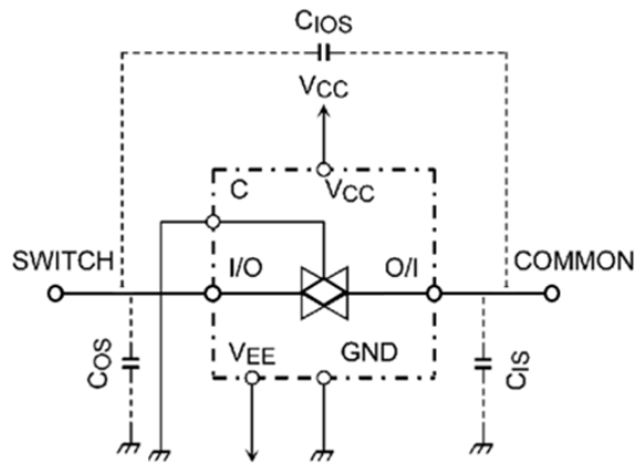
図2. C_{ios} , C_{is} , C_{os}
