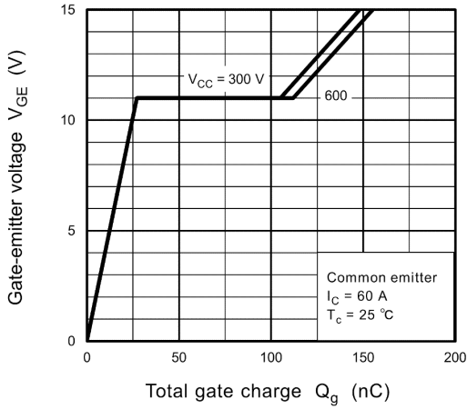
Fig. 8.7 V_{GE} - Q_g
