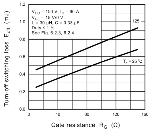
Fig. 8.16 E_{off} - R_G
