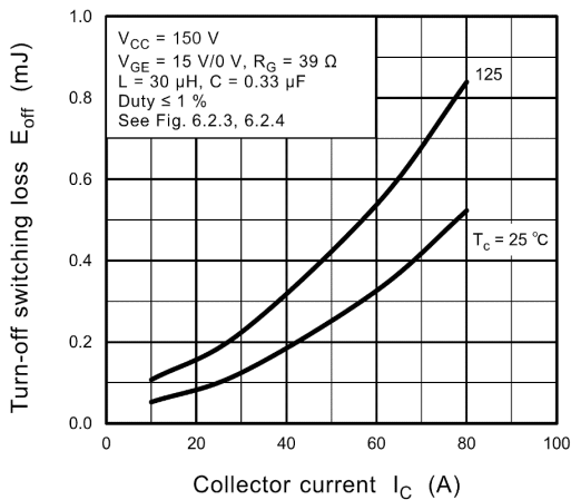
Fig. 8.15 E_{off} - I_C
