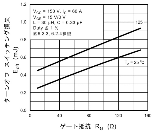
図 8.16 E_{off} - R_G
