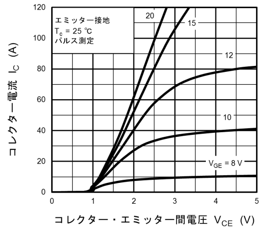
図 8.2 I_C - V_{CE}
