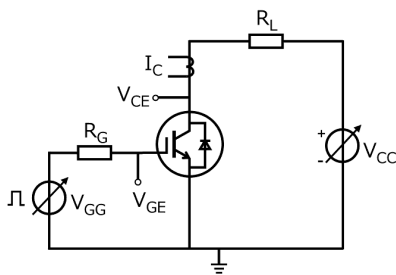
図 6.2.1 スwitchング時間の測定回路
