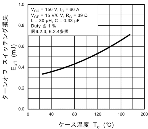
図 8.17 E_{off} - T_c
