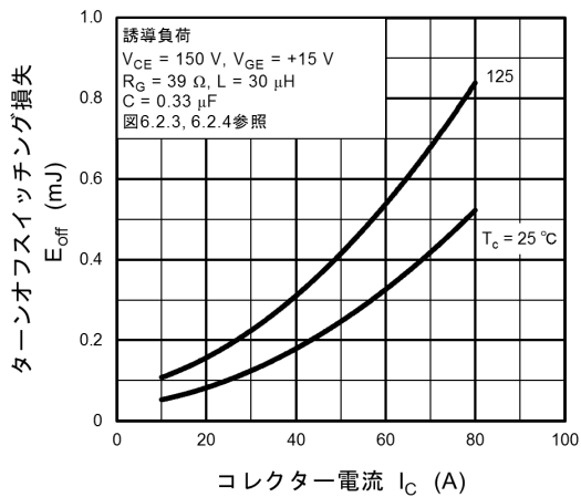
図 8.15 E_{off} - I_C
