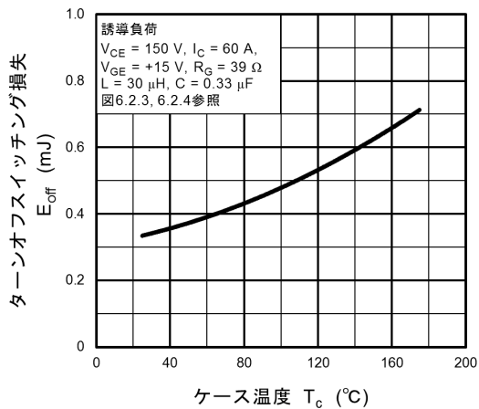
図 8.17 E_{off} - T_C
