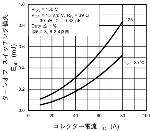
図 8.15 E_{off} - I_c
