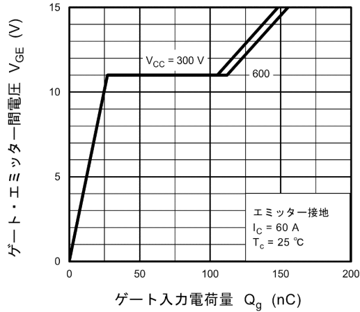
図 8.7 V_{GE} - Q_g
