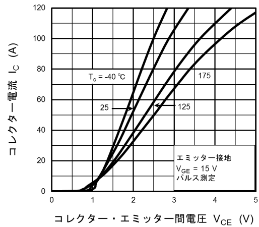
図 8.4 I_C - V_{CE}
