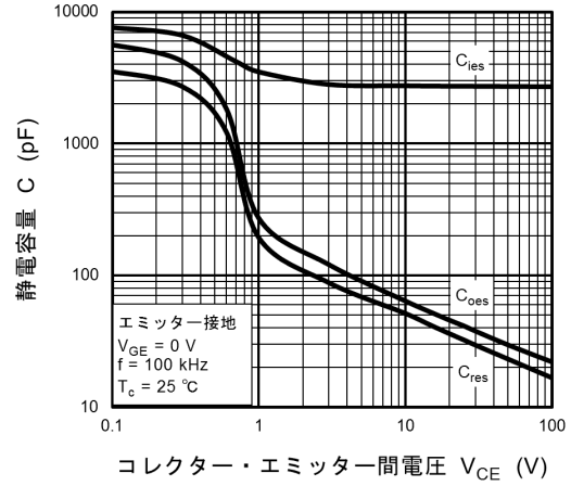
図 8.8 C - V_{CE}
