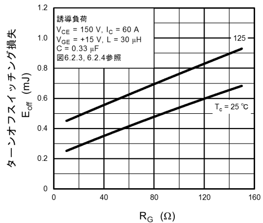
図 8.16 E_{off} - R_G
