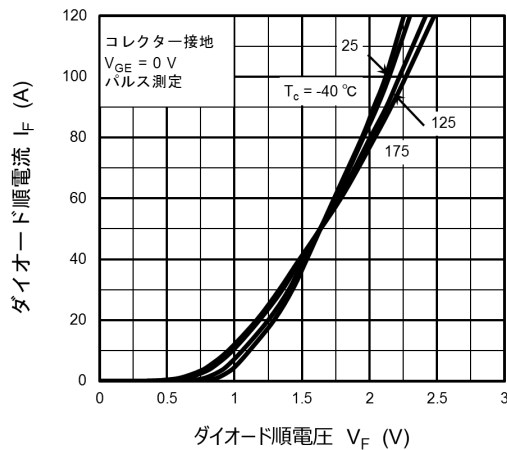
図 8.11 I_F - V_F
