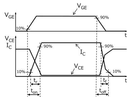
図 6.2.2 スwitchング時間のタイミングチャート
