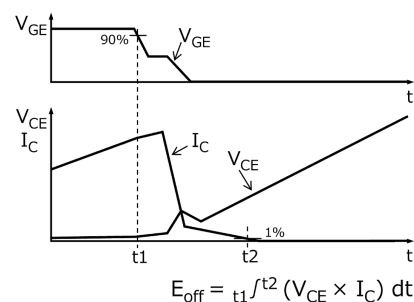
図 6.2.4 スwitchング損失のタイミングチャート
