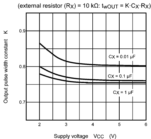
図 16.3 出力パルス幅定数K - 電源電圧 (標準) (外付け抵抗 ( R_X ) = 10 k\Omega : t_{wOUT} = K \cdot C_X \cdot R_X )
