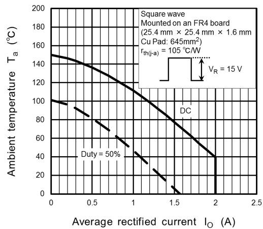
Fig. 9.6 T_a - I_O
