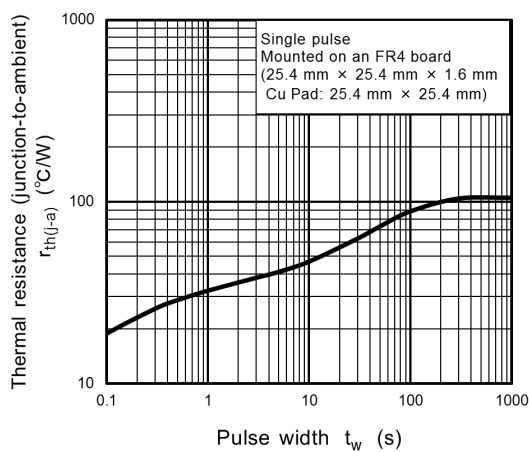
図 9.4 r_{th} - t_w
