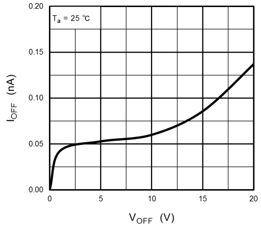
I_{OFF} - V_{OFF}
