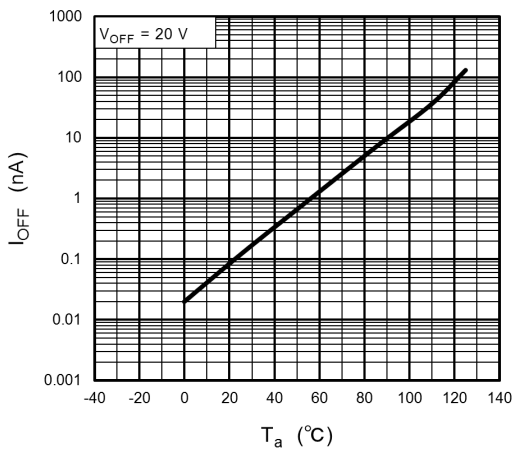
Fig. 12.8 I_{OFF} - T_a
