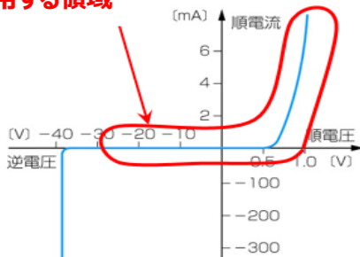
スイッチングダイオードの電流vs電圧特性
