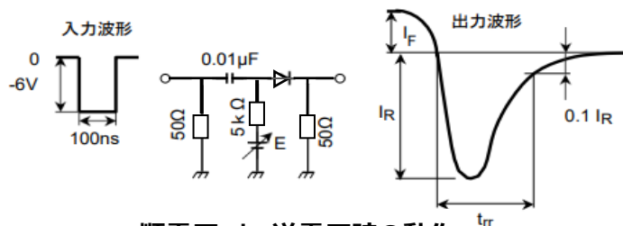
順電圧 と 逆電圧時の動作
