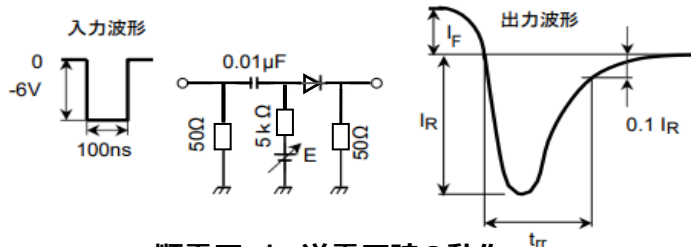
順電圧 と 逆電圧時の動作
