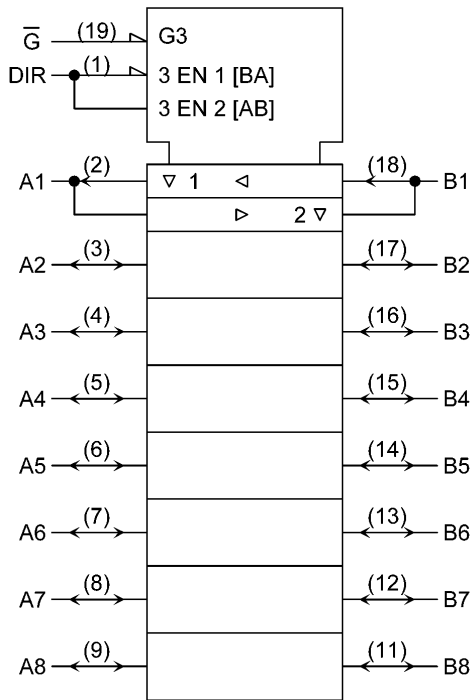
TC74AC245F
