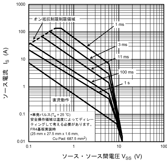
図 9.9 安全動作領域
