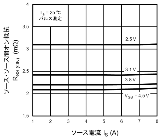
図 9.2 R_{SS(ON)} - I_S
