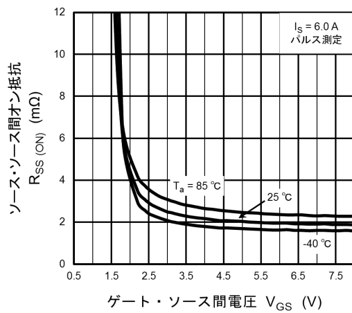
図 9.4 R_{SS(ON)} - V_{GS}
