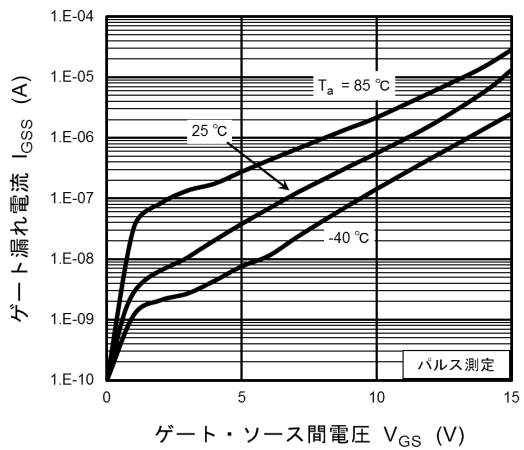
図 9.6 I_{GSS} - V_{GS}
