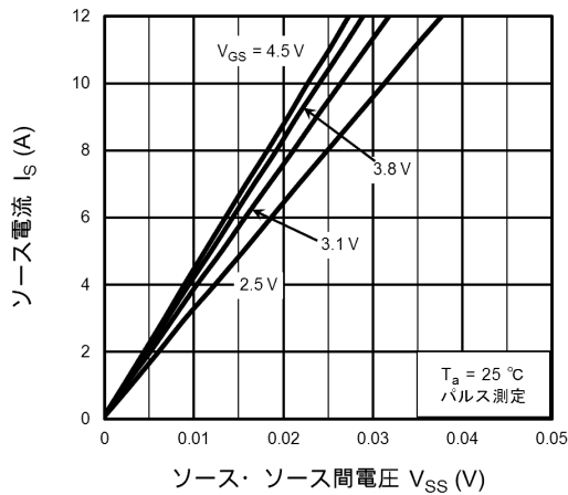
図 9.1 I_S - V_{SS}
