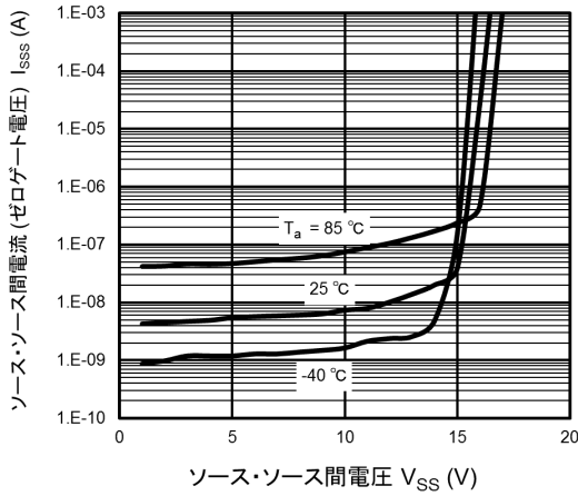
図 9.7 I_{SSS} - V_{SS}
