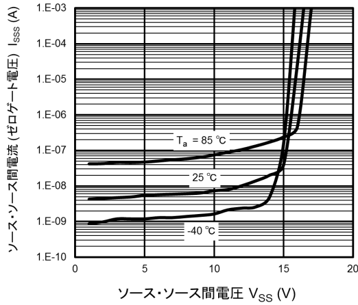
図 9.7 I_{SSS} - V_{SS}
