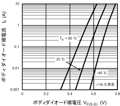
図 9.5 I_F - V_F
