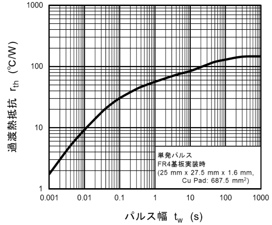
図 9.8 r_{th} - t_w
