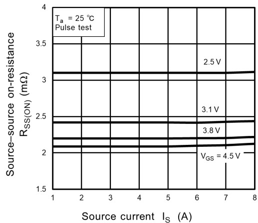
Fig. 9.2 R_{SS(ON)} - I_S
