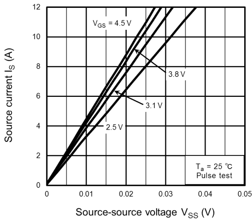
Fig. 9.1 I_S - V_{SS}
