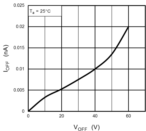
Fig. 12.9 I_{OFF} - V_{OFF}
