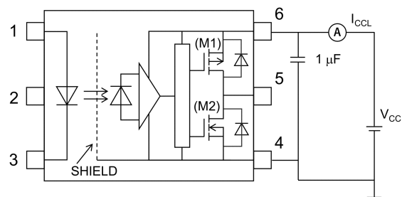
図 13.1.6 I CCL 測定回路
