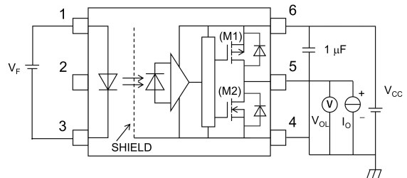
図 13.1.4 V OL 測定回路
