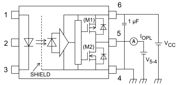
図 13.1.2 I OPL 測定回路
