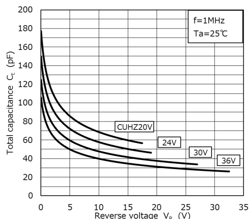
C_t - V_R (2)
