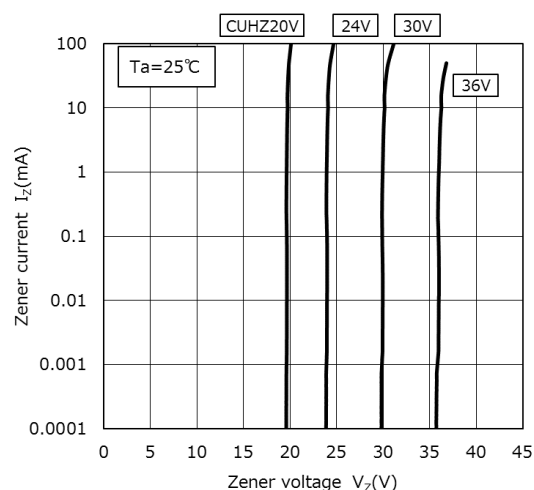
I_Z - V_Z (2)
