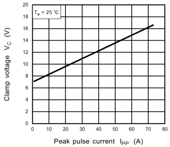
V_C - I_{PP} (注 2)
