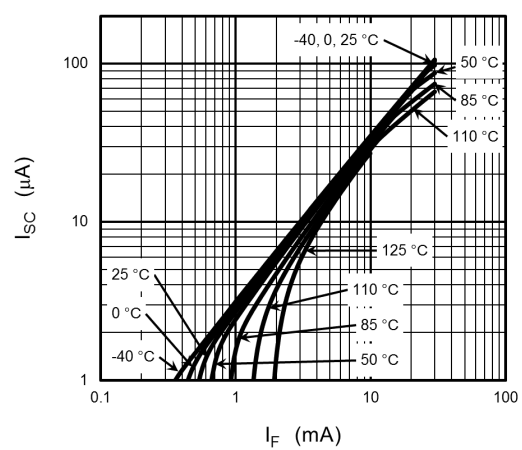
図 12.6 I_{SC} - I_F
