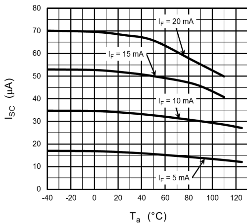
図 12.9 I_{SC} - T_a
