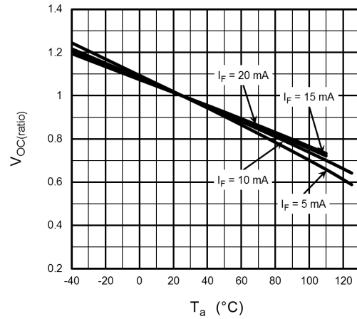
図 12.8 V_{OC}(\text{ratio}) - T_a
