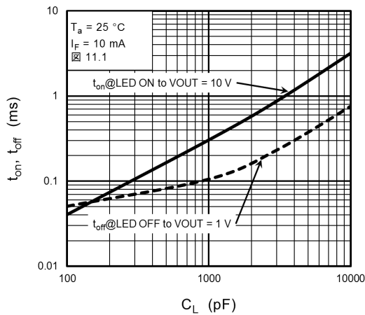
図 12.11 t_{on}, t_{off} - C_L
