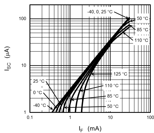
図 12.6 I_{SC} - I_F
