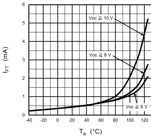
図 12.3 I_{FT} - T_a
