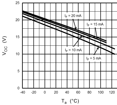
図 12.7 V_{OC} - T_a
