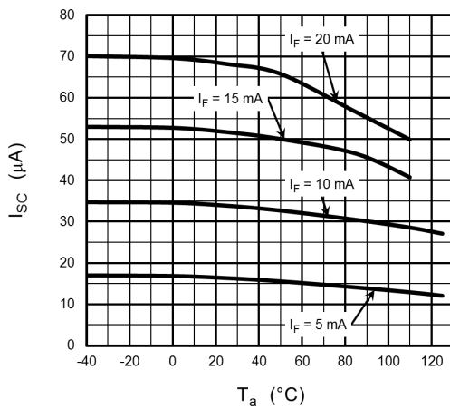
図 12.9 I_{SC} - T_a
