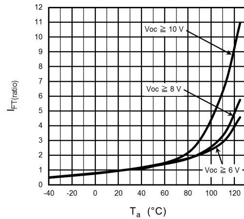
図 12.4 I_{FT}(\text{ratio}) - T_a
