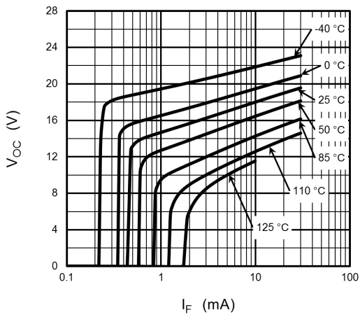
図 12.5 V_{OC} - I_F
