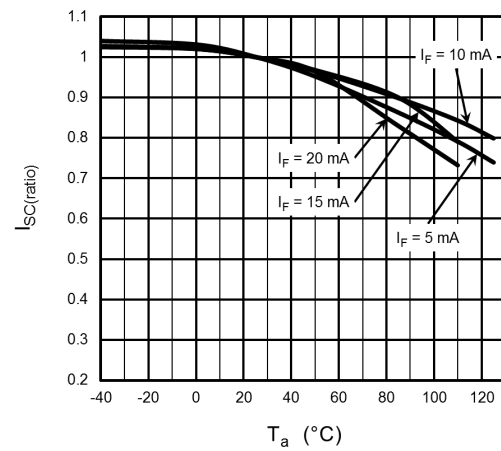
図 12.10 I_{SC}(\text{ratio}) - T_a
