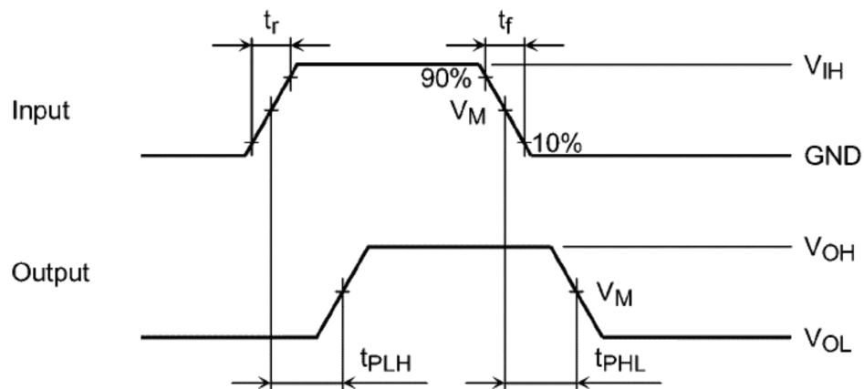
図 12.6.1 t PLH , t PHL
