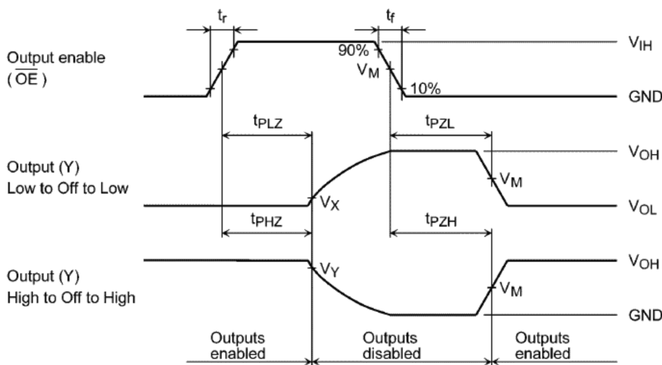
図 12.6.2 t PLZ , t PHZ , t PZL , t PZH
