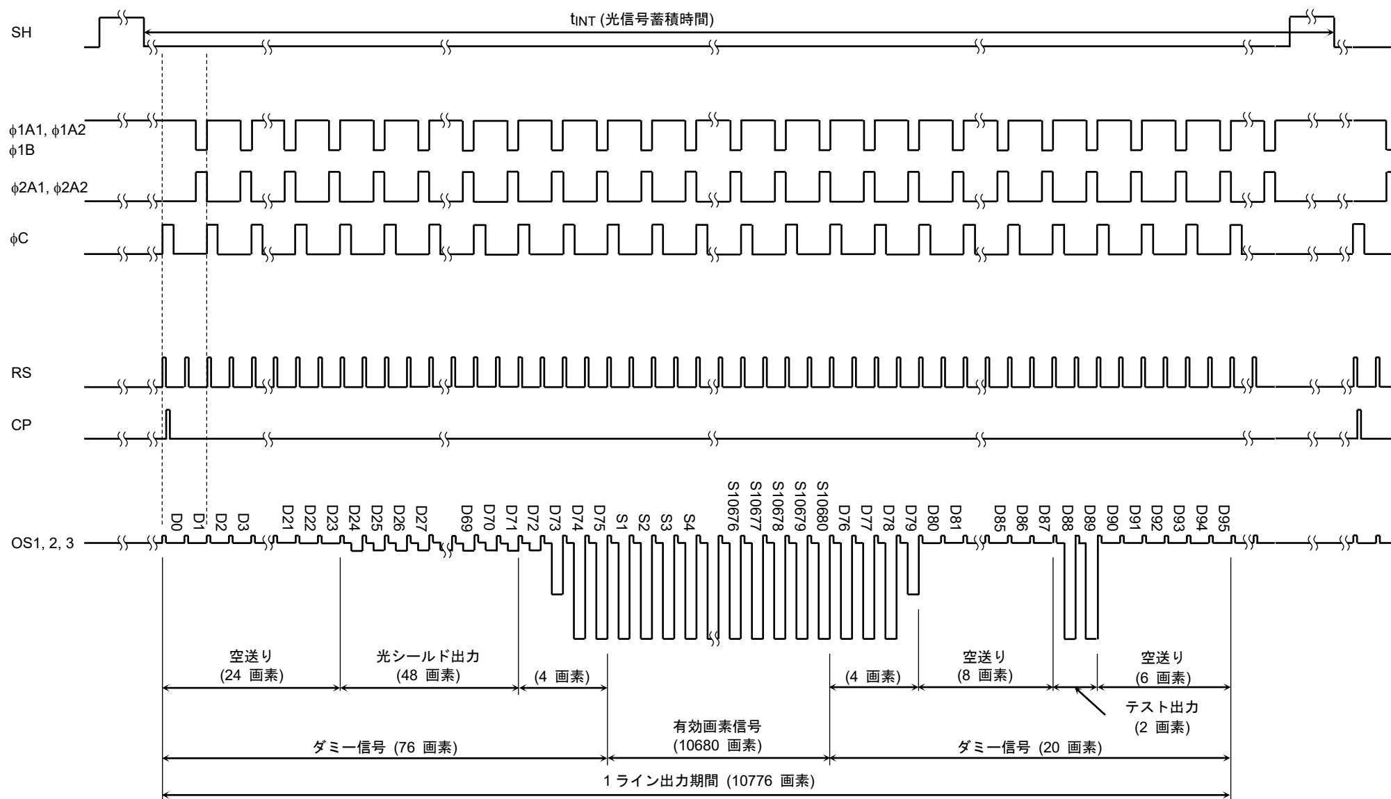
タイミング図 2: 1200 dpi モード (ラインクランプモード)
