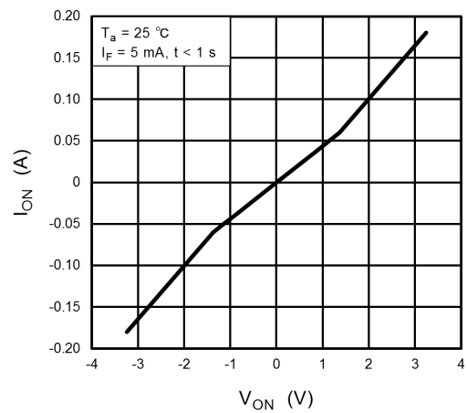
Fig. 12.4 I_{ON} - V_{ON}
