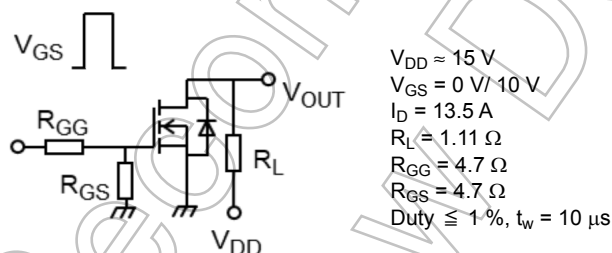
図 6.2.1 スwitchング時間の測定回路図
