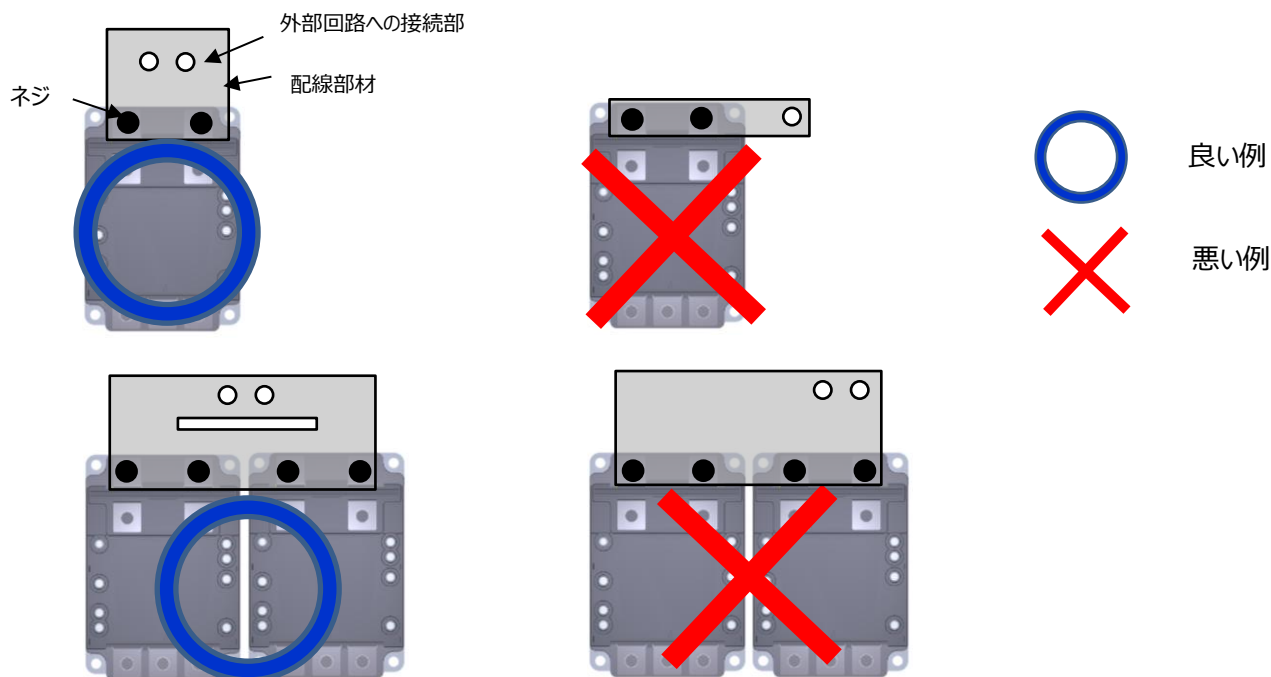
図 2.5.2 端子と主回路配線部材の設計例(P 端子の接続例)
