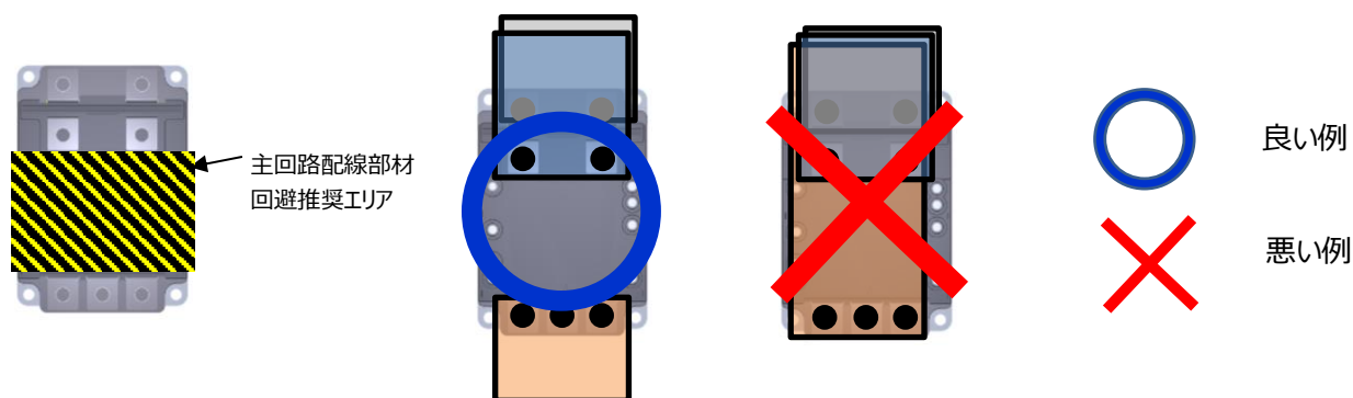
図 2.5.3 主回路配線部材の設計例(N-AC 端子間の取り回し例)
