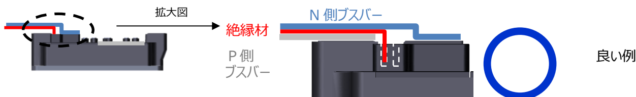
図 2.5.4 P-N 主回路配線部材の推奨平行配線・絶縁例
