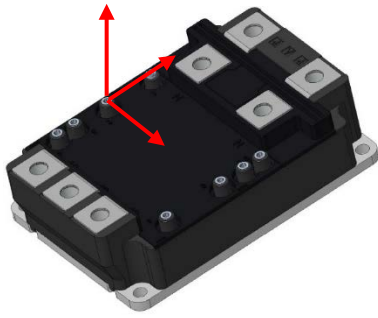
図 2.6.1 端子 1~8 への信号回路配線部材の取り付け時の最大許容荷重
