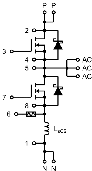
図 1.2.1 回路構成
