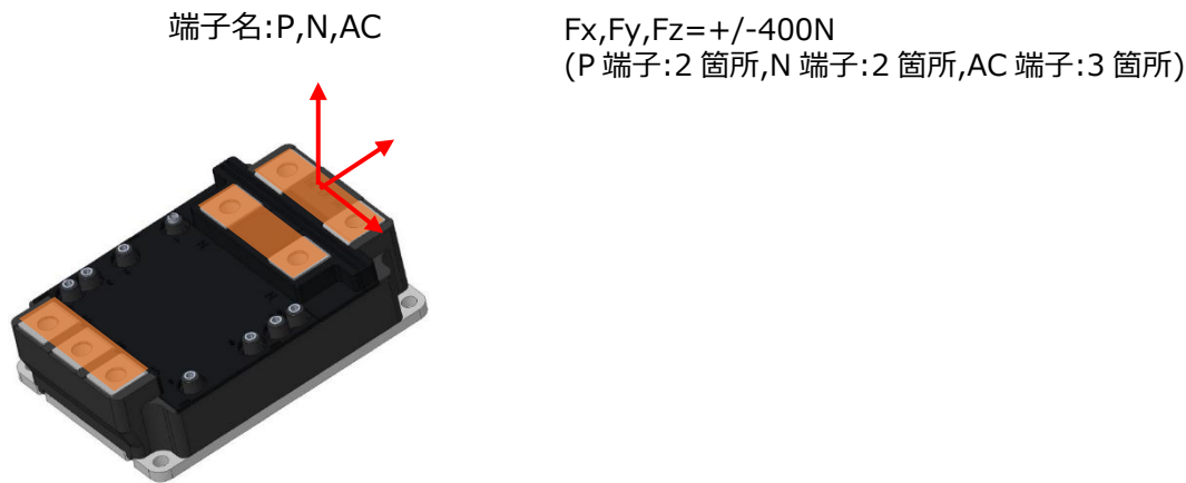
図 2.5.8 P,N,AC 端子の主回路配線部材の取り付け時の最大許容荷重
