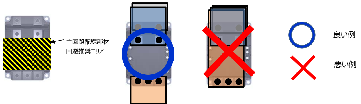
図 2.5.3 主回路配線部材の設計例(N-AC 端子間の取り回し例)
