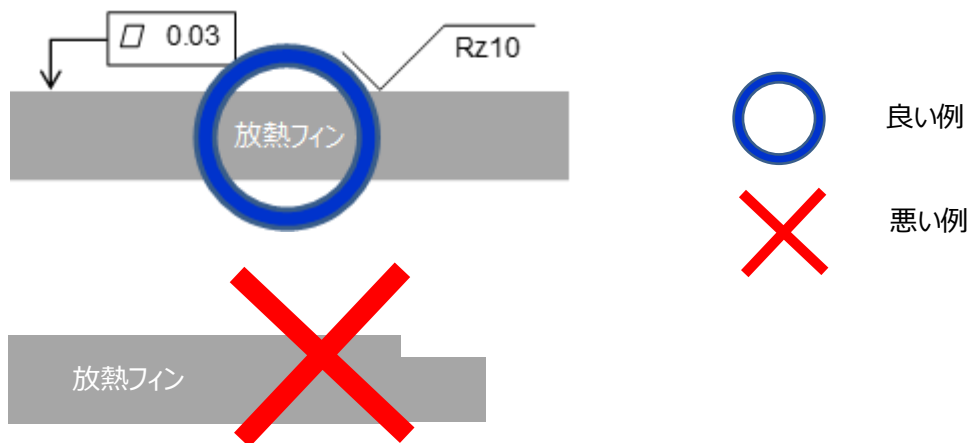
図 2.4.2.1 放熱フィンの平面度、面粗さ
