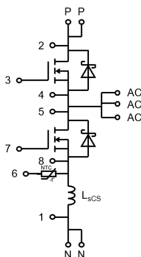
図 1.2.1 回路構成
