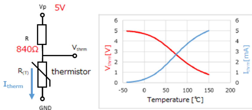
図 1.3.2 サーミスターの温度検出の回路と出力電圧、電流の例
