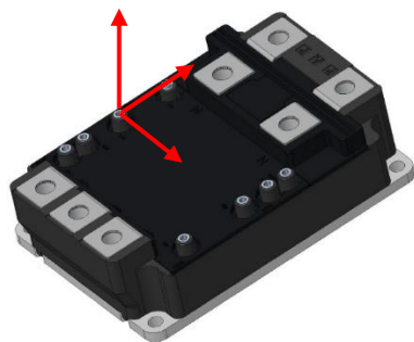
図 2.6.1 端子 1~8 への信号回路配線部材の取り付け時の最大許容荷重
