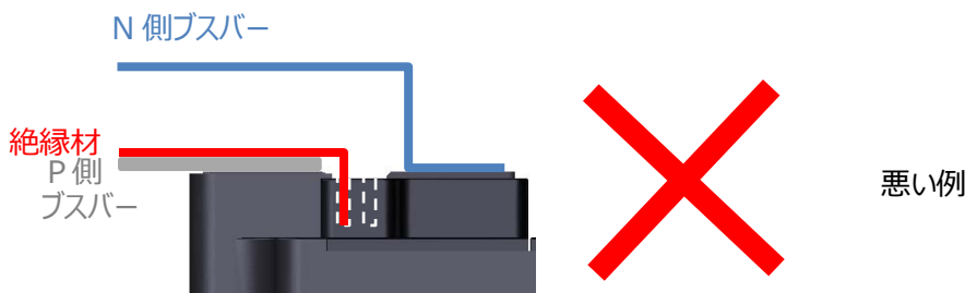
図 2.5.5 P-N 主回路配線部材の間隔をあけることにより、主回路インダクタンスが増加する例
