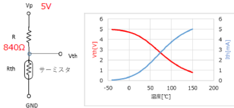
図 1.3.2 サーミスタの温度検出の回路と出力電圧、電流の例
