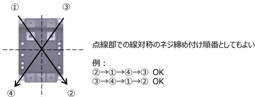
図 2.4.4.1 放熱フィンと素子間のネジ締め付け順番
