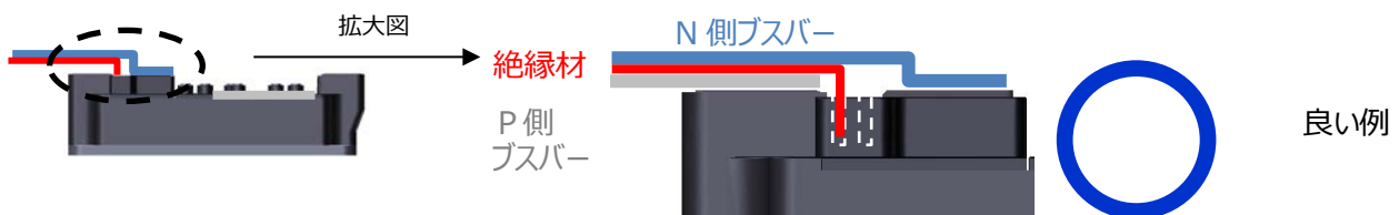
図 2.5.4 P-N 主回路配線部材の推奨平行配線・絶縁例
