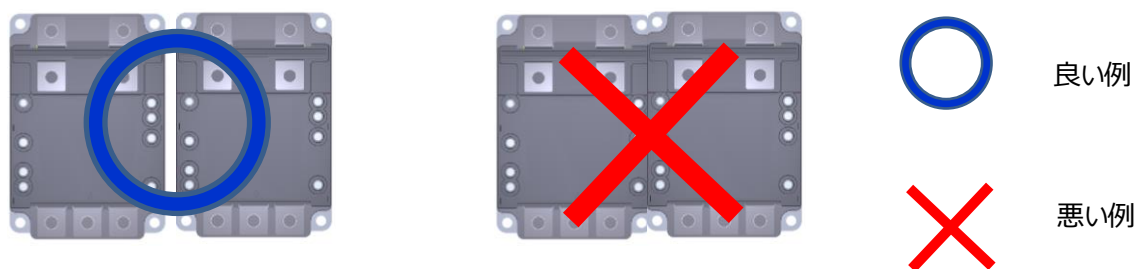
図 2.4.1.1 放熱フィンに複数の素子を取り付ける際の注意事項
