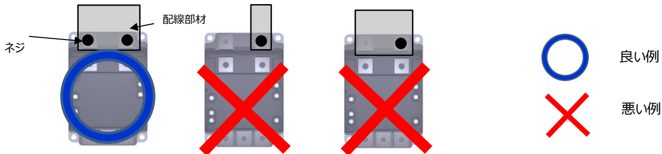
図 2.5.1 端子と主回路配線部材の接続(P 端子の接続例)
