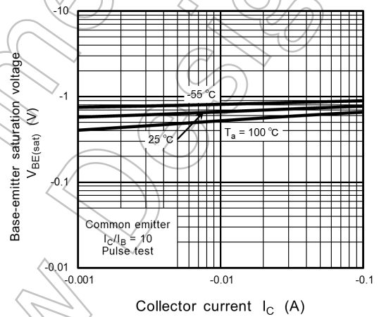
Fig. 7.4 V_{BE(sat)} - I_C
