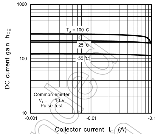
Fig. 7.2 h_{FE} - I_C
