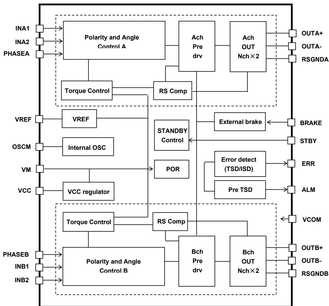
図 3.1 ブロック図
