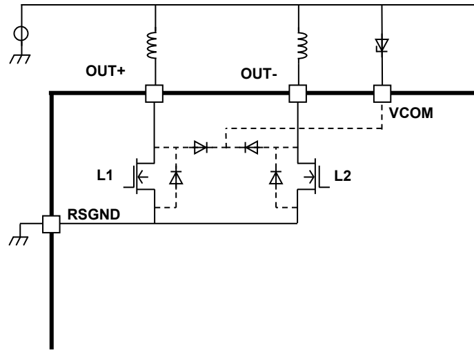
図 6.9 MOSFET 同時オン防止機能等価回路
