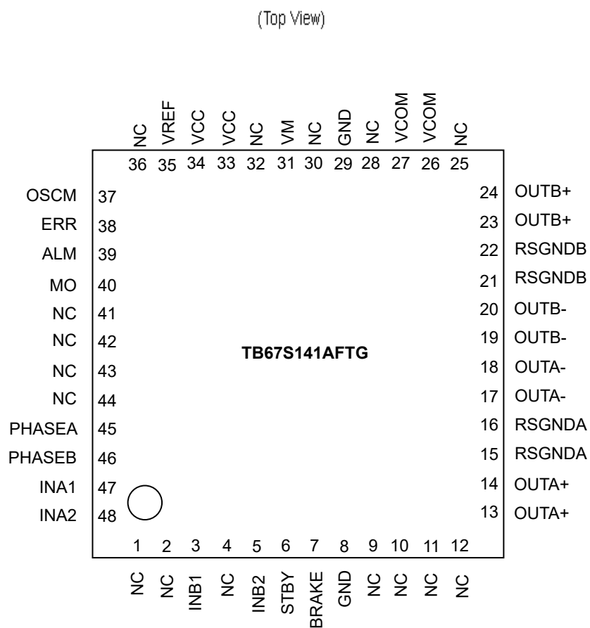
图 4.1 端子配置图
