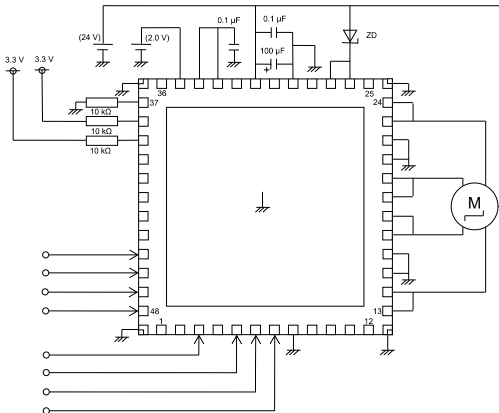
図 10.1 応用回路例
