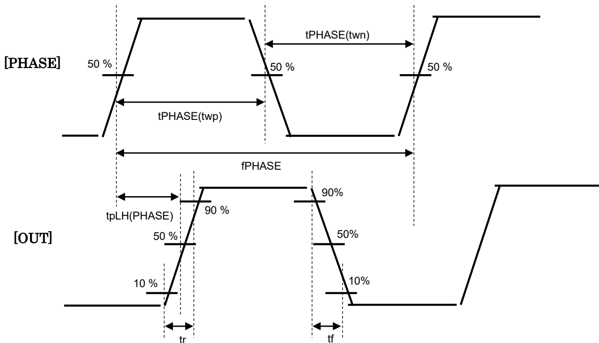
図 9.1 AC 特性タイミングチャート
