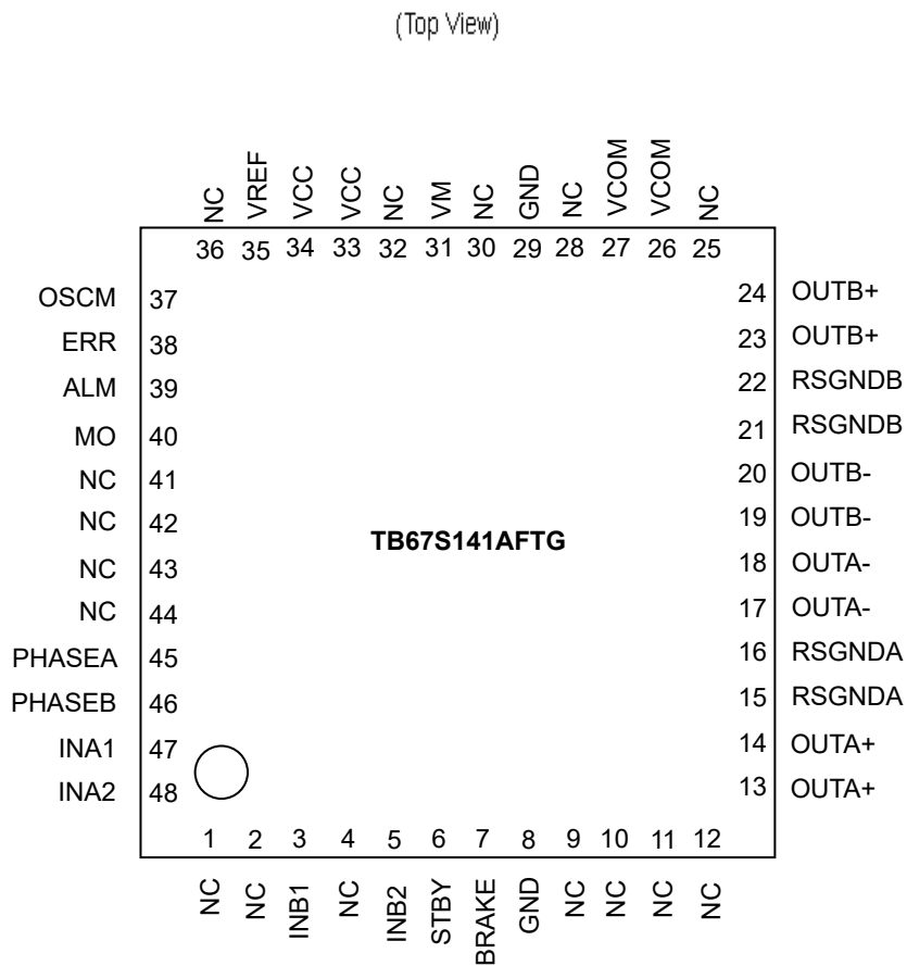
图 4.1 端子配置图
