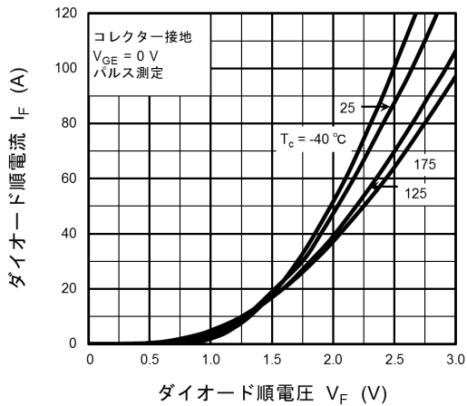
図 8.11 I_F - V_F
