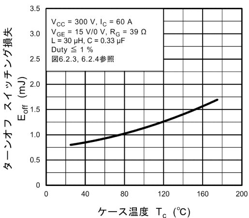
図 8.17 E_{\text{off}} - T_c
