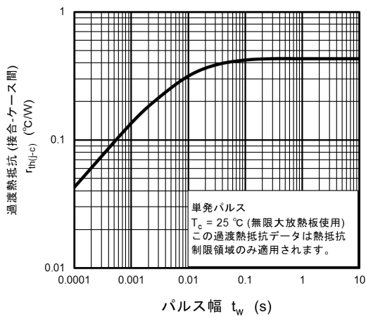
図 8.9 r_{th(j-c)} - t_w (最大値 (保証値))
