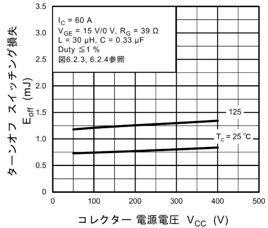
図 8.14 E_{\text{off}} - V_{CC}
