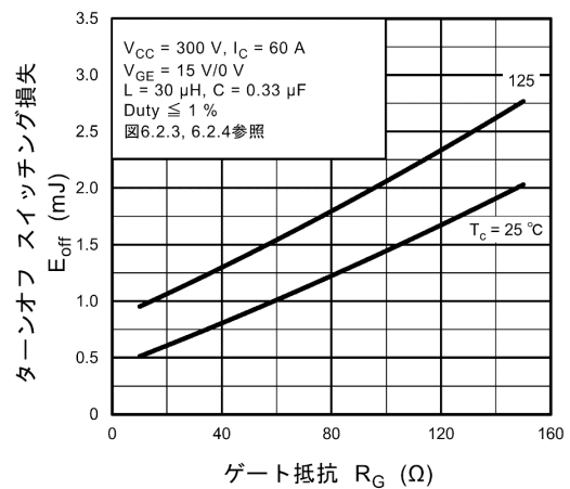
図 8.16 E_{\text{off}} - R_G
