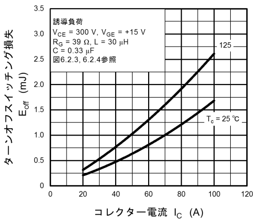
図 8.15 E_{off} - I_C
