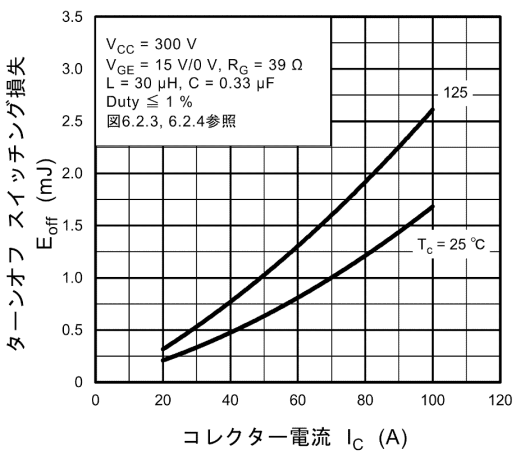
図 8.15 E_{off} - I_C
