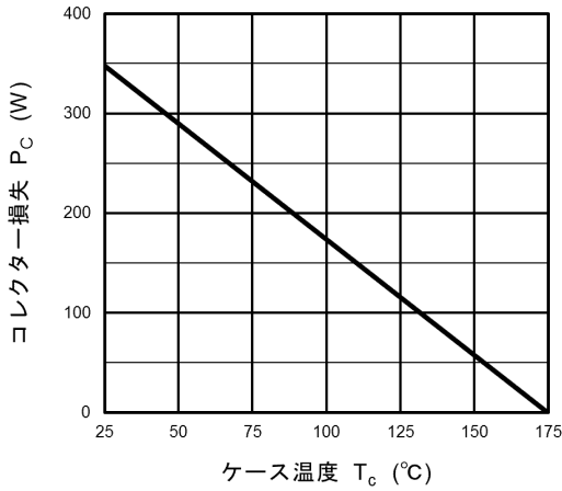
図 8.13 P_C - T_c
