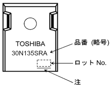
図 7.1 現品表示
