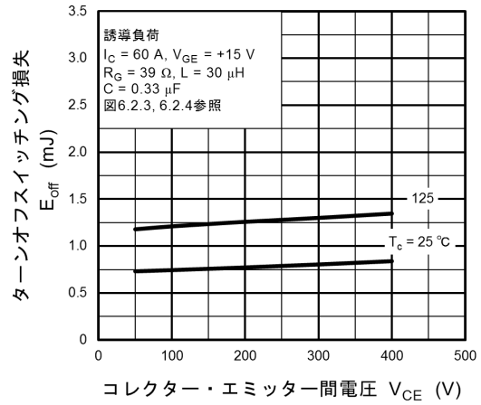
図 8.14 E_{off} - V_{CE}
