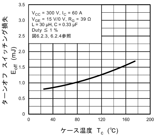
図 8.17 E_{off} - T_c
