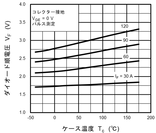
図 8.12 V_F - T_c
