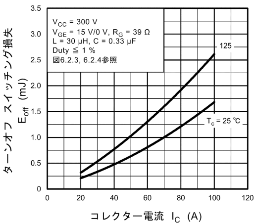
図 8.15 E_{\text{off}} - I_C
