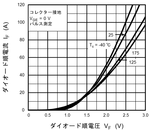
図 8.11 I_F - V_F
