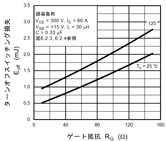
図 8.16 E_{off} - R_G
