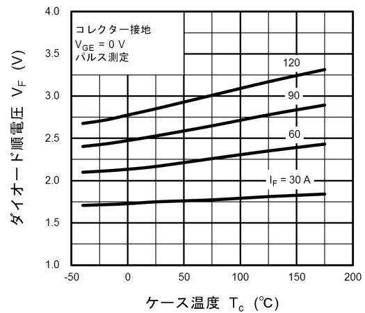
図 8.12 V_F - T_c
