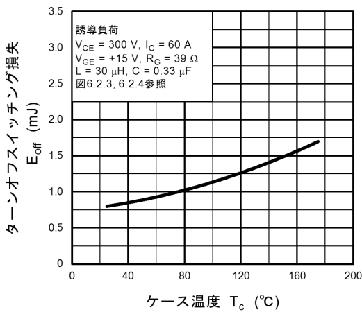
図 8.17 E_{off} - T_c
