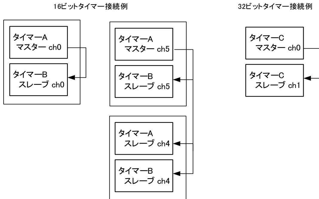
図 3.4 同期動作例
