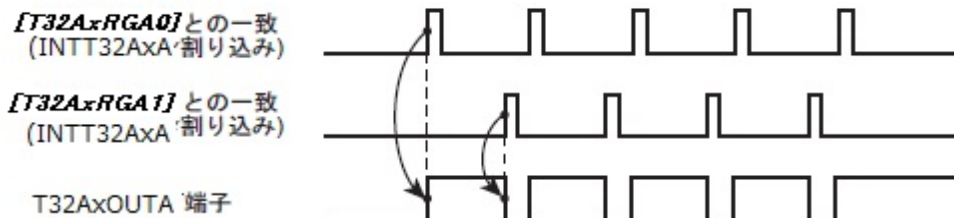
図 3.5 16ビットタイマーAを使用したプログラマブル矩形波出力例
