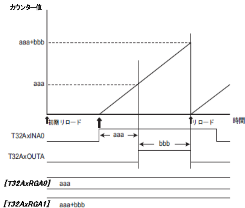
図 5.6 外部トリガーによるPPG出力例
