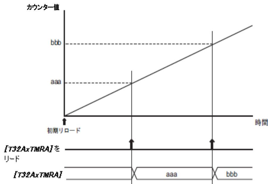
図 5.3 イベントカウンター例
