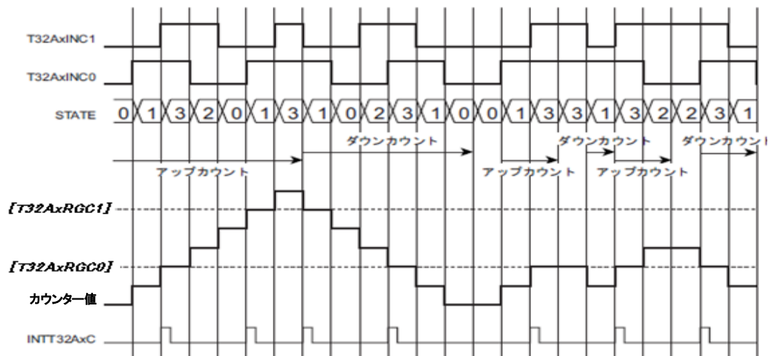
図 3.2 正位相(<PDIR>=0)時のカウンター動作例
