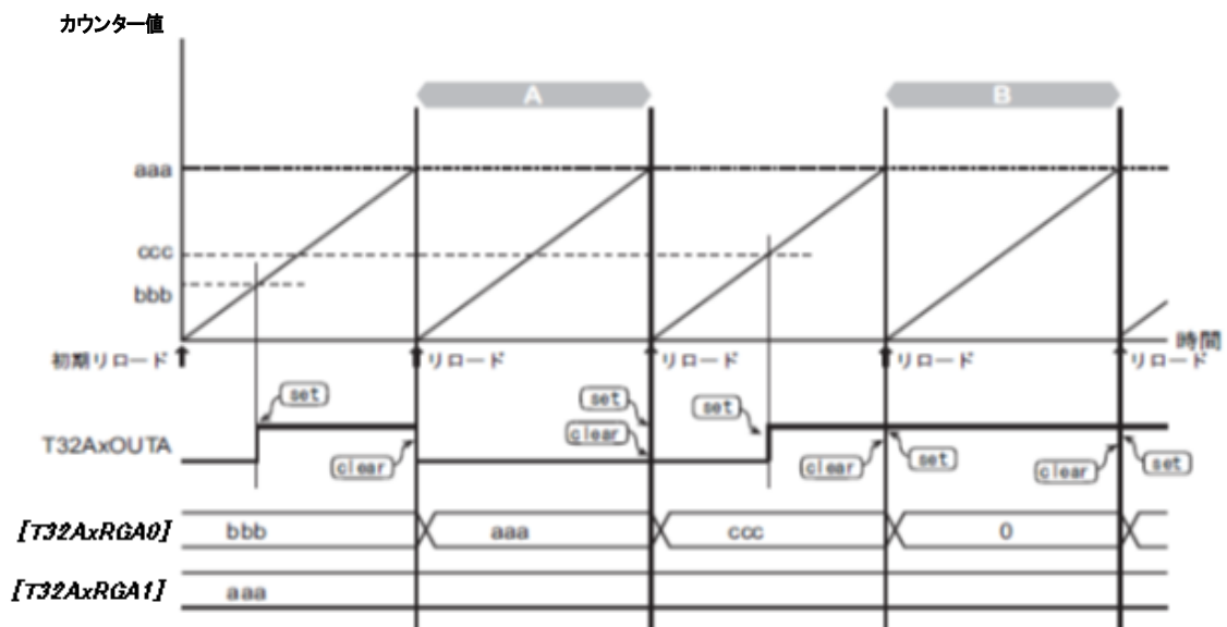
図 5.5 PPG出力 (期間A,Bの場合の動作例)
