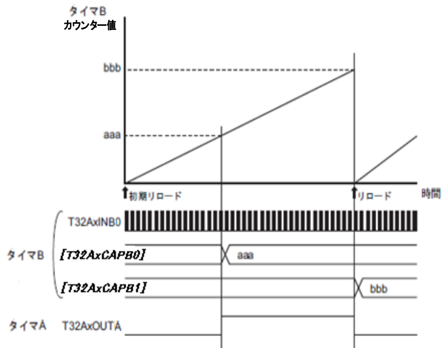
図 5.9 キャプチャーを利用した周波数測定例
