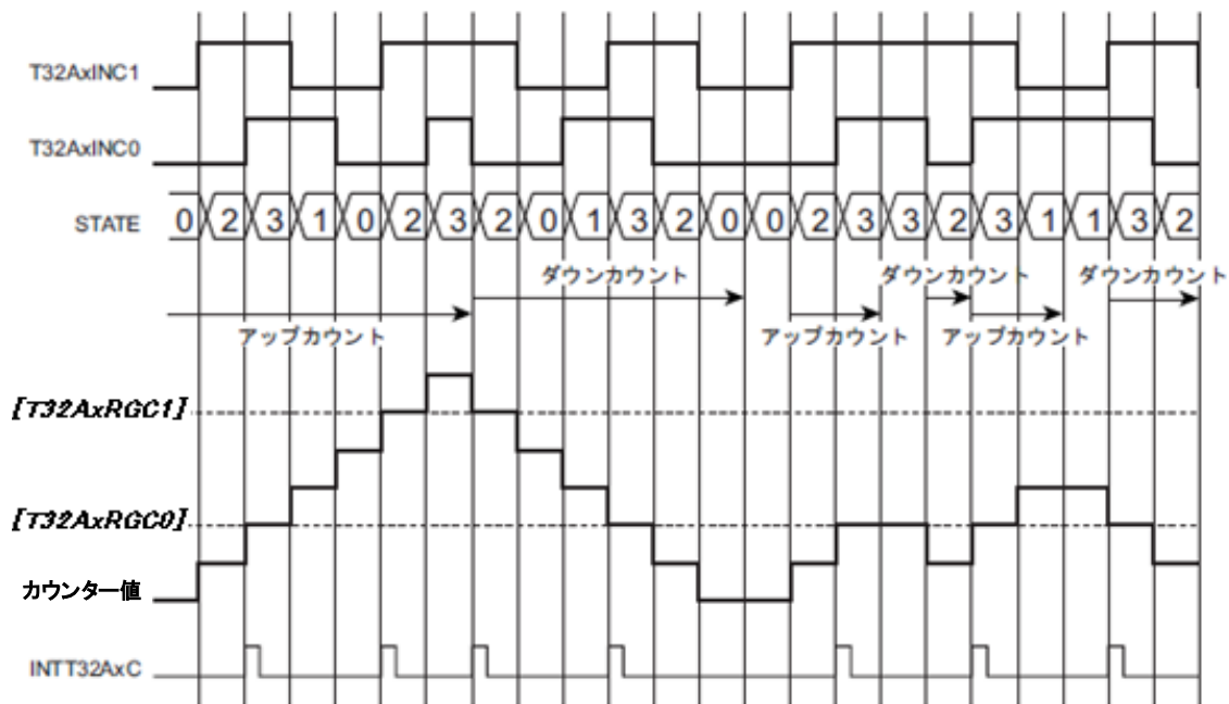
図 3.3 逆位相(<PDIR>=1)時のカウンター動作例
