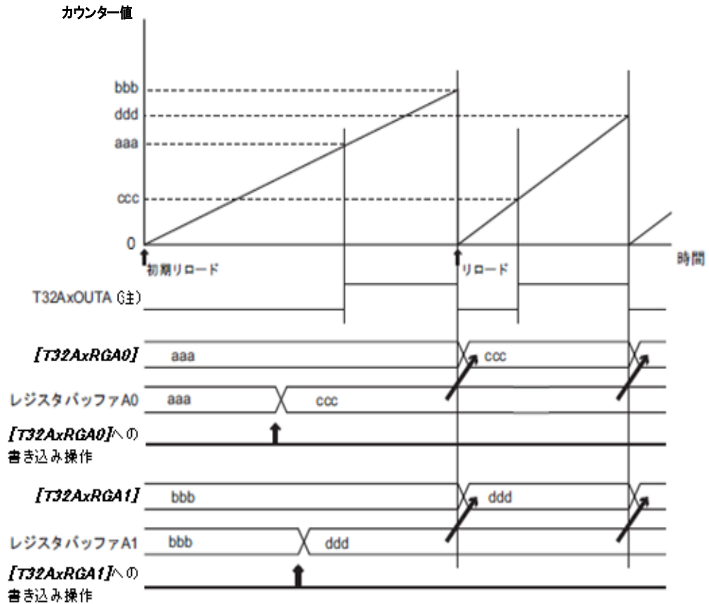
図 5.4 PPG出力例 (Lowアクティブ)
