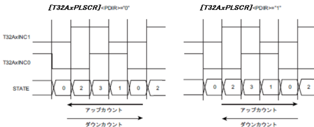
図 3.1 状態遷移
