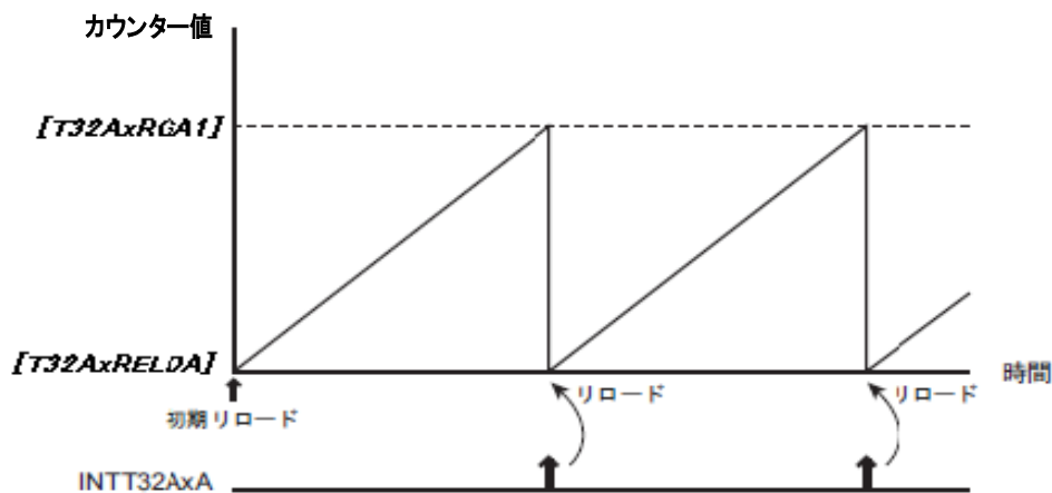
図 5.1 インターバルタイマー例 (アップカウント)
