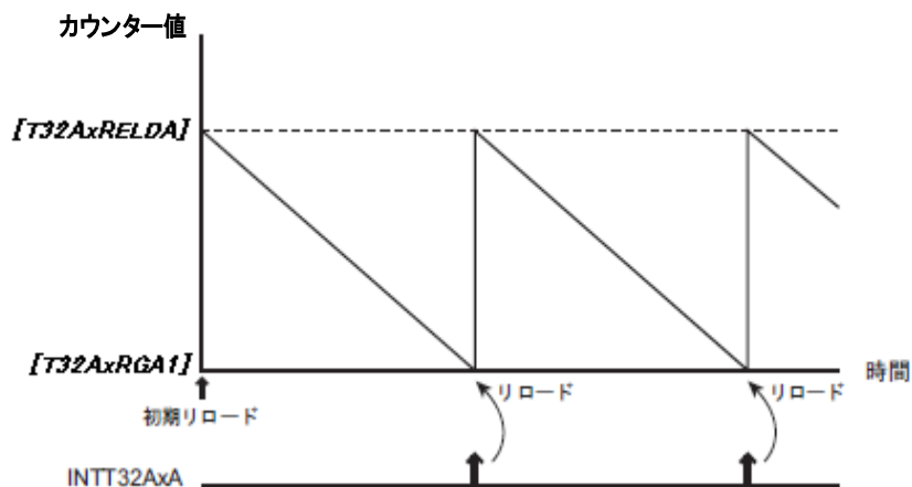
図 5.2 インターバルタイマー例 (ダウンカウント)
