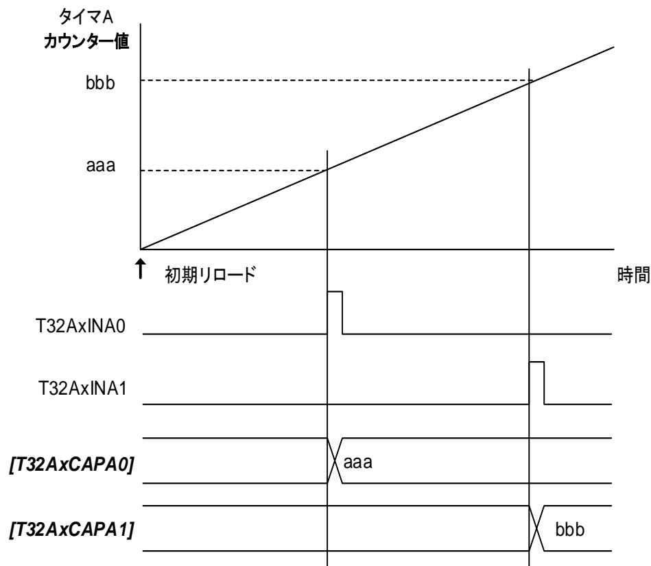
図 5.11 キャプチャーを利用した時間差測定例
