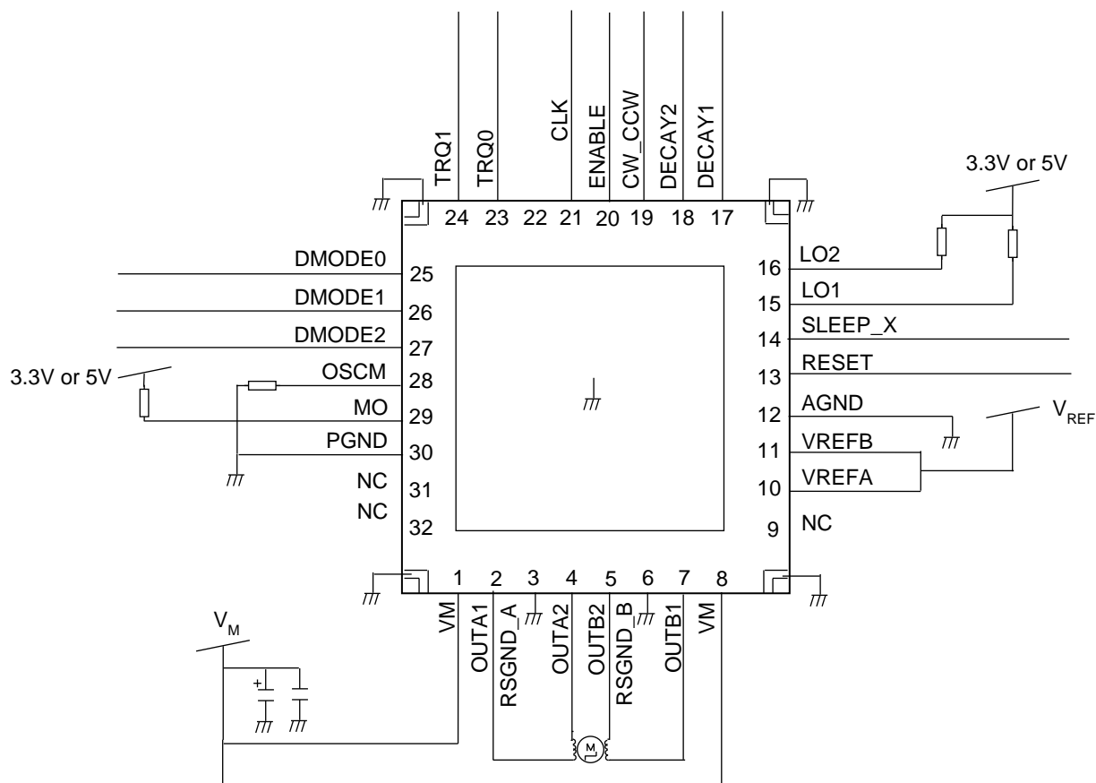
図 10 応用回路例
