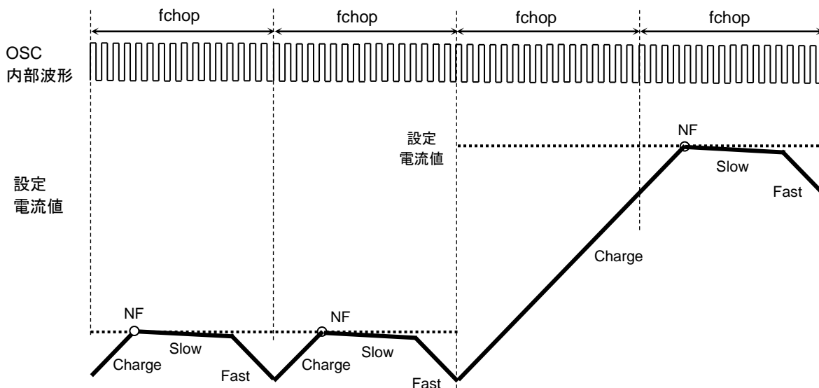
図 6.13 Charge 期間が f_{chop} 1 周期以上の場合
