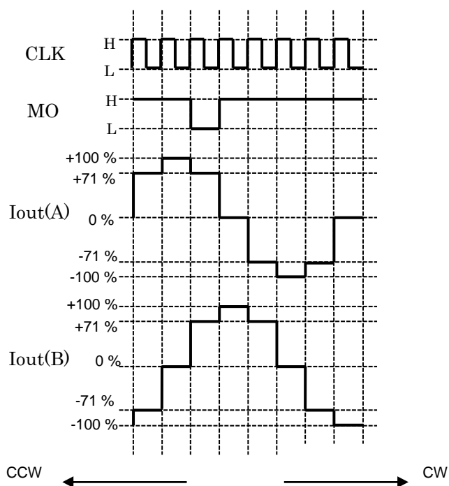
図 6.2 1-2 相励磁(B タイプ)設定
