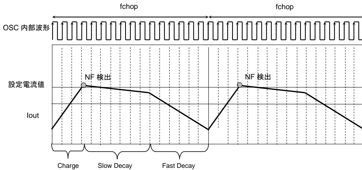
図 6.9 Mixed Decay の波形
