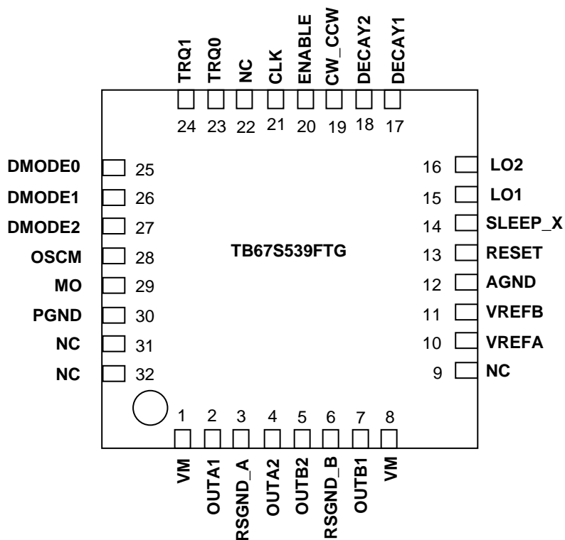
图 4.1 端子配置图
