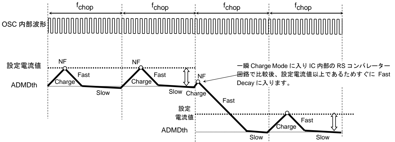
図 6.20 設定電流値が減少方向の場合
