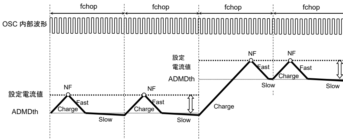
図 6.18 設定電流値が増加方向の場合
