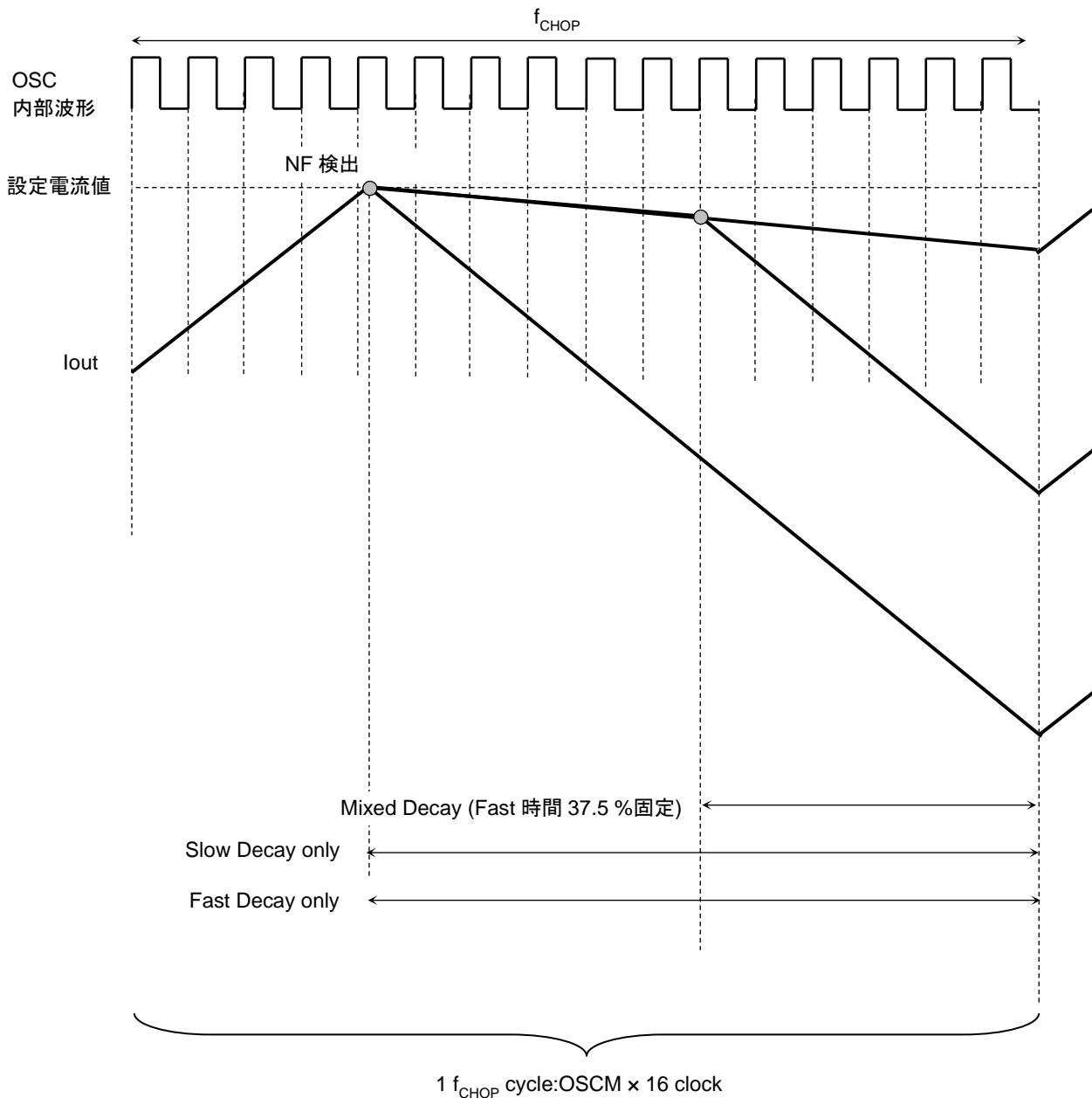
図 6.8 Selectable Mixed Decay ファンクション
