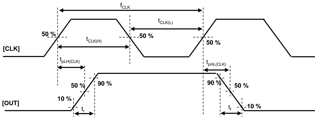
図 9.1 TB67S539FTG(CLK と出力の関係)
