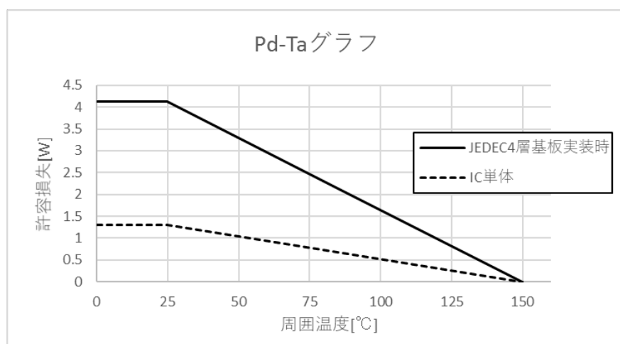
図 7.1 PD-Ta グラフ
