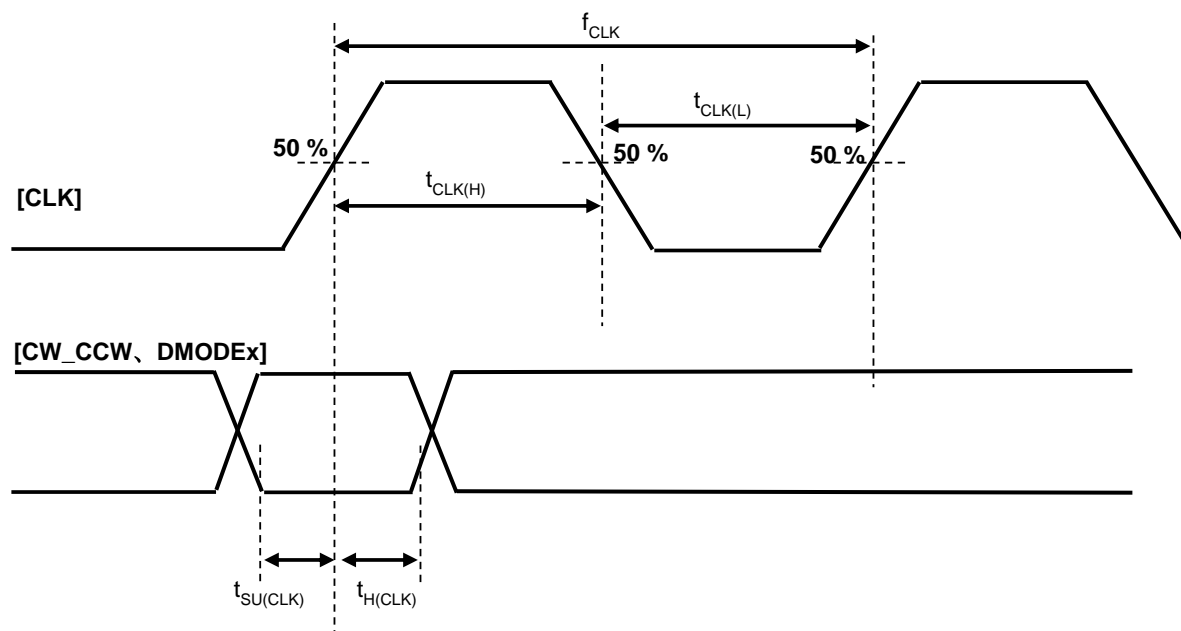
図 9.2 TB67S539FTG(CLK とその他制御信号の関係)
