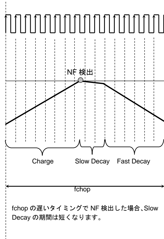
図 6.11 定電流 PWM 動作の各時間 (2)
