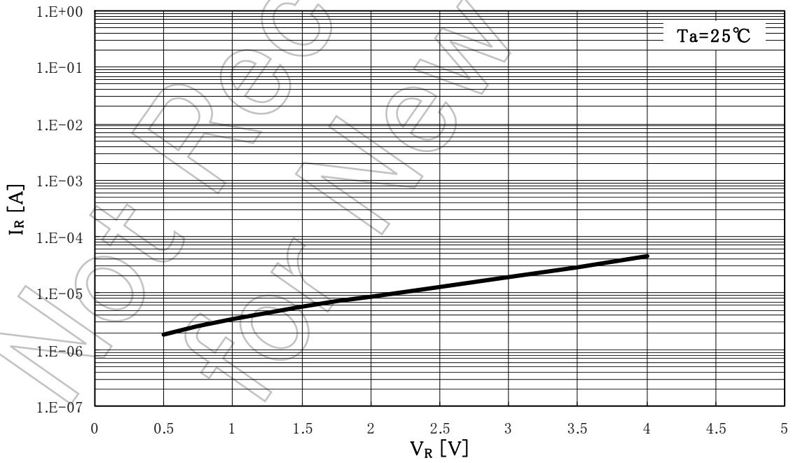
I_R - V_R
