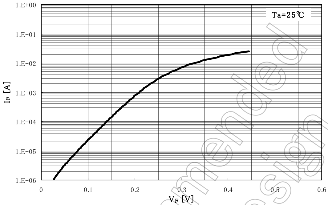
I_F - V_F
