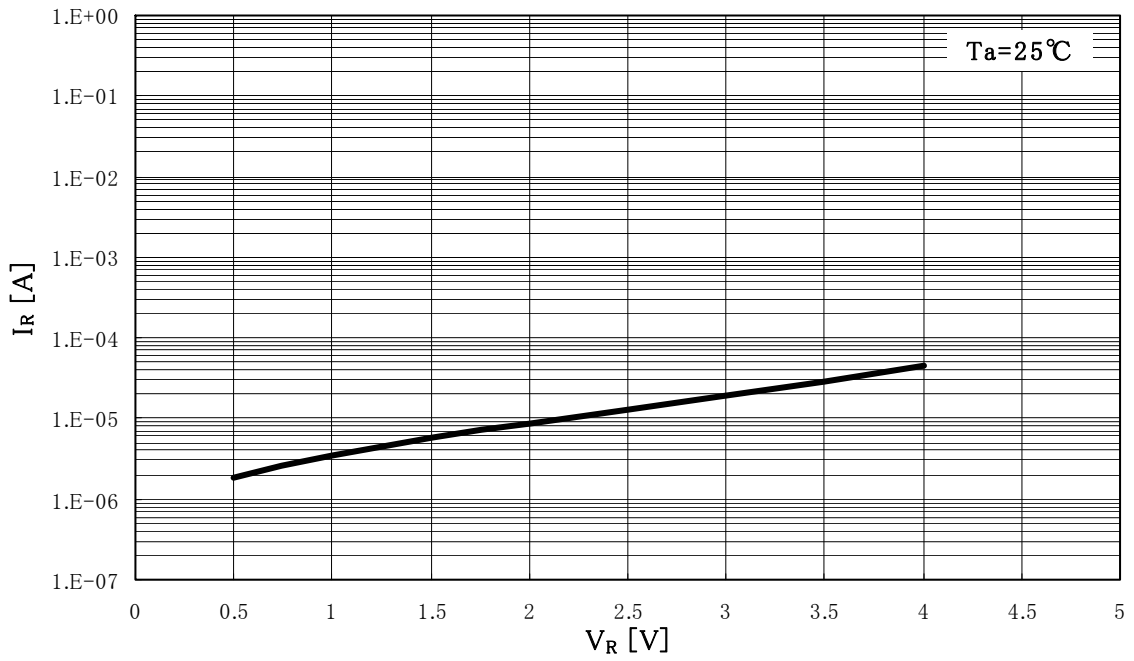
I_R - V_R
