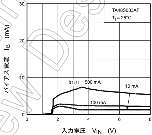
I_B - V_{IN}
