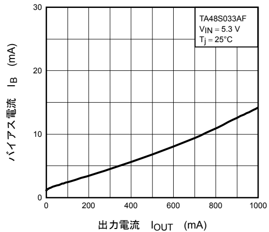
I_B - I_{OUT}
