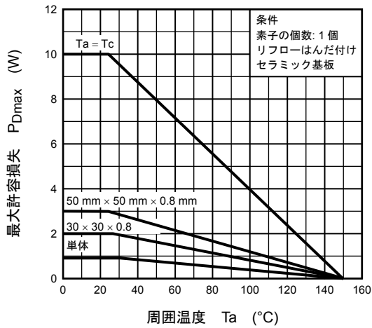
P_{Dmax} - T_a
