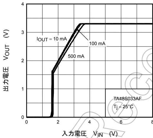
V_{OUT} - V_{IN}
