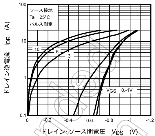
I_{DR} - V_{DS}
