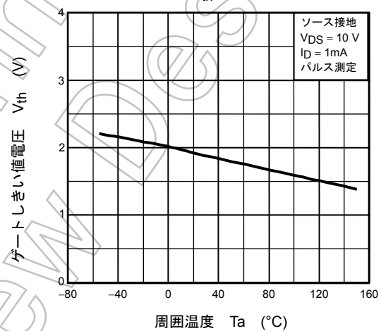
V_{th} - T_a
