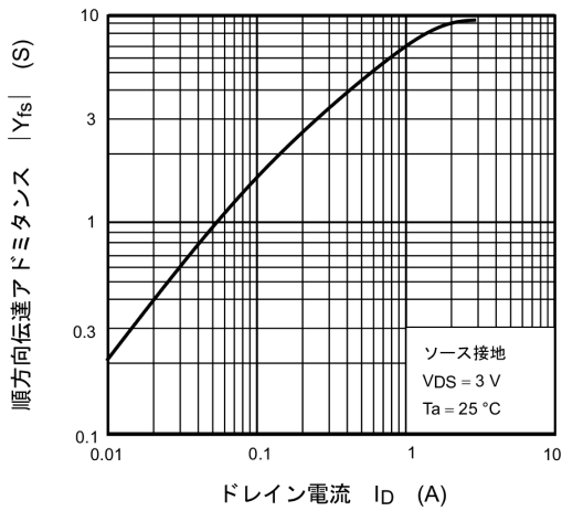
図 7.7 |Y_{fs}| - I_D
