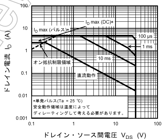
図 7.12 安全動作領域
