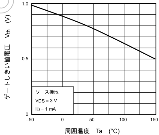
図 7.6 V_{th} - T_a
