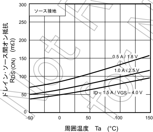
図 7.5 R_{DS(ON)} - T_a
