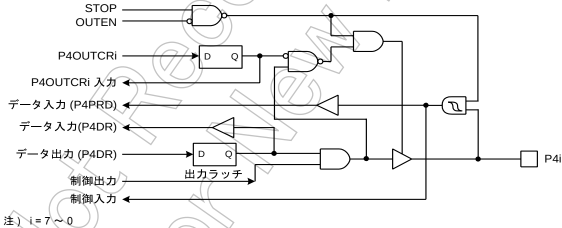
図 5-6 P4 ポート
