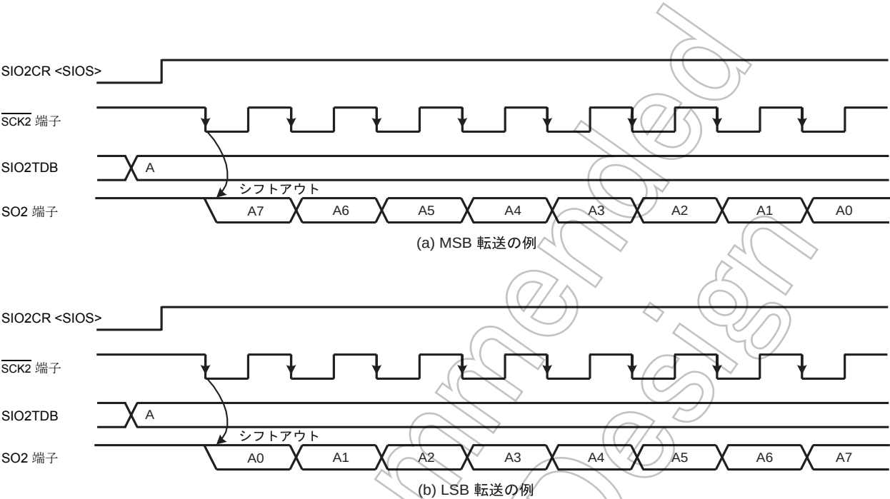
図 15-5 転送ビット方向 ( 送信モードの例 )
