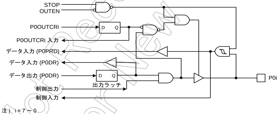
図 5-2 P0 ポート
