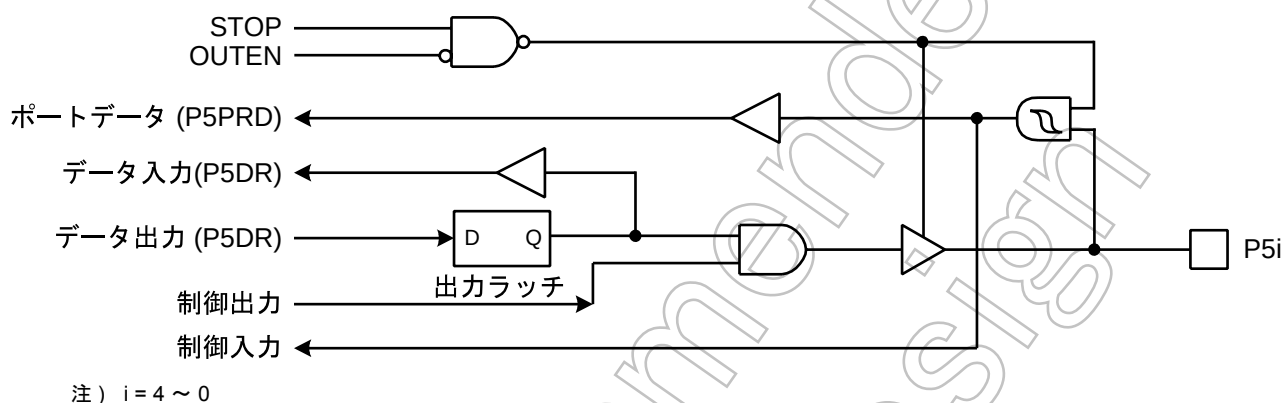
図 5-7 P5 ポート
