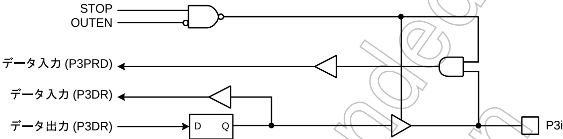
図 5-5 P3 ポート
