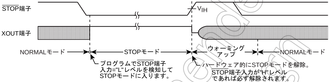
図 2-7 レベル解除モード
