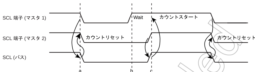
図 16-4 クロック同期化の例
