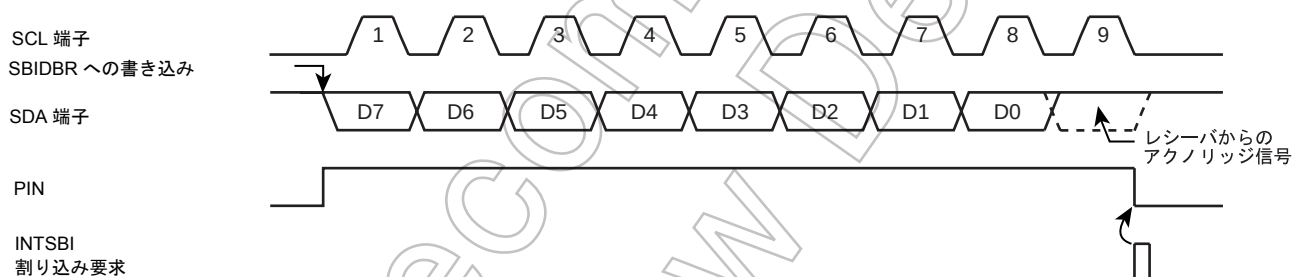
図 16-10 BC="000", ACK="1" の場合
