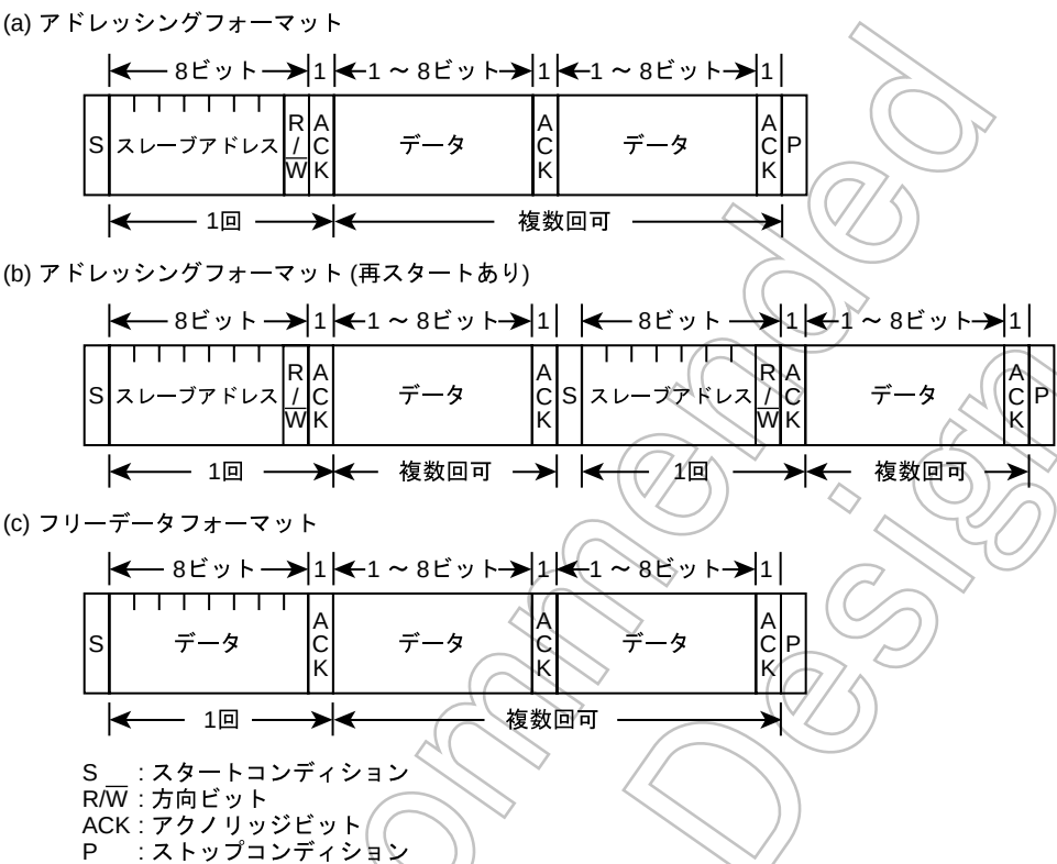
図 16-2 I 2 C バスのデータフォーマット
