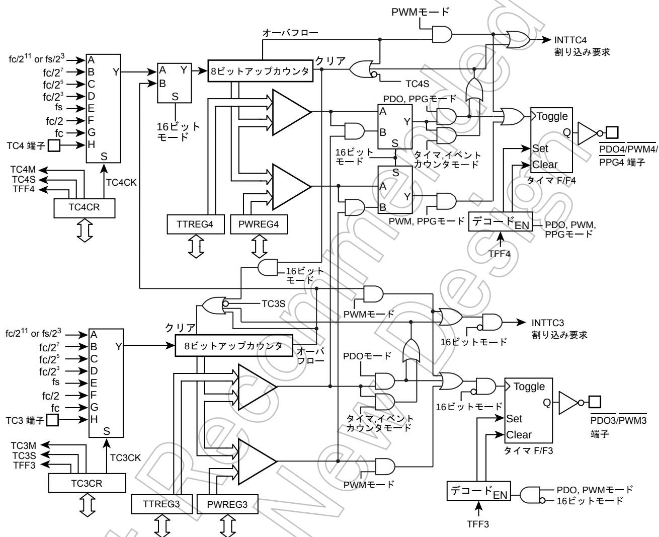
図 10-1 8 ビットタイマカウンタ 3, 4
