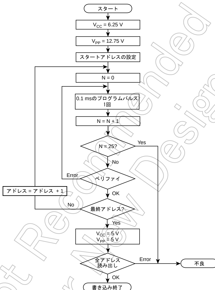
図 19-3 書き込みフローチャート
