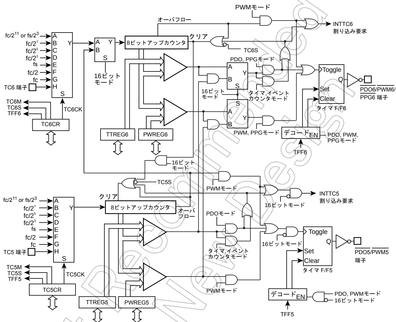
図 11-1 8 ビットタイマカウンタ 5, 6
