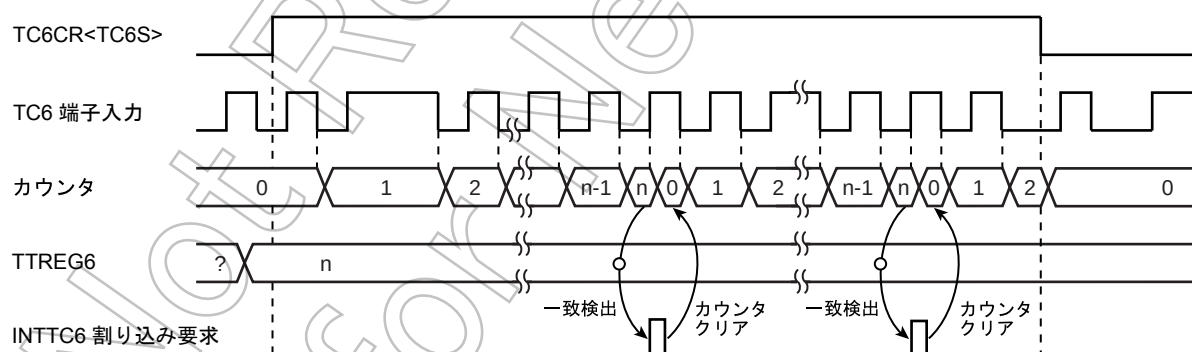
図 11-3 8 ビットイベントカウンタモードタイミングチャート (TC6 の場合)
