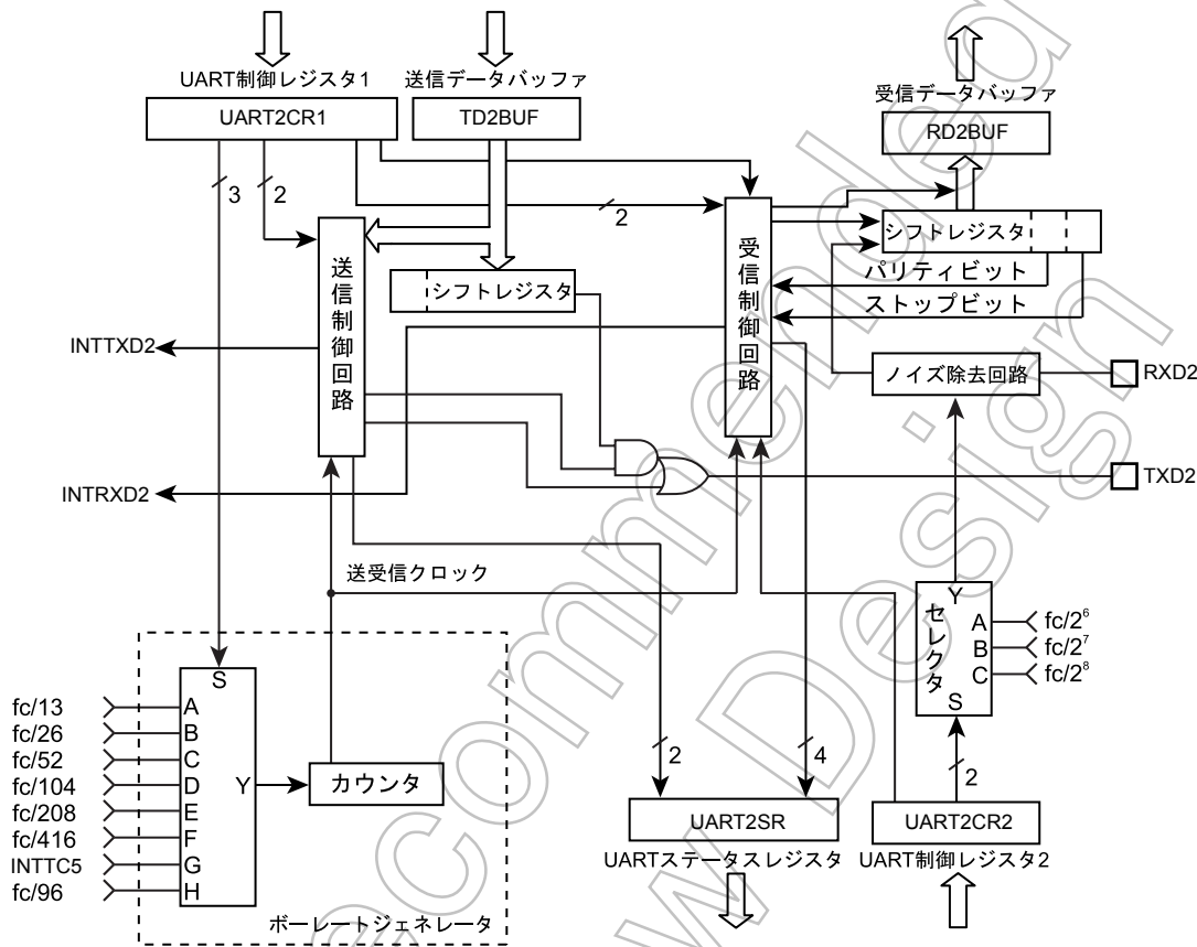
図 13-1 UART2 ( 非同期型シリアルインタフェース )
