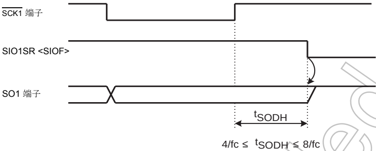
図 14-8 送信終了時のデータ保持時間
