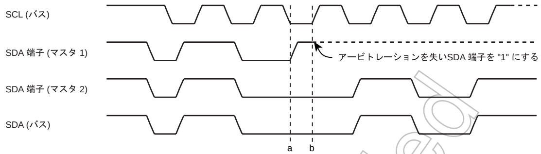
図 16-7 アービトレーションロスト
