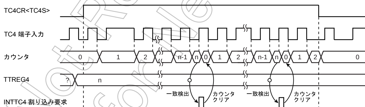
図 10-3 8 ビットイベントカウンタモードタイミングチャート (TC4 の場合)
