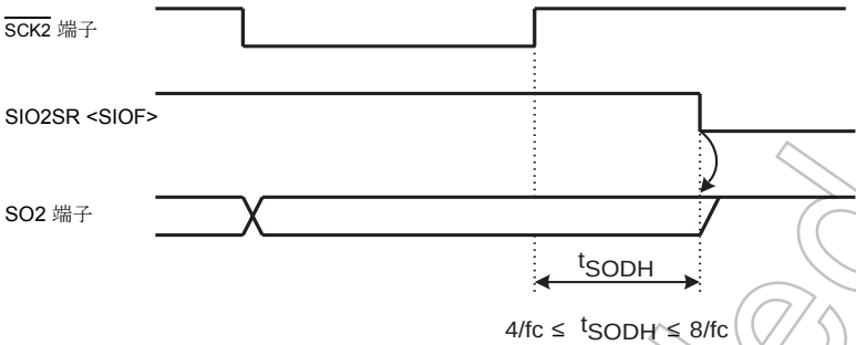
図 15-8 送信終了時のデータ保持時間
