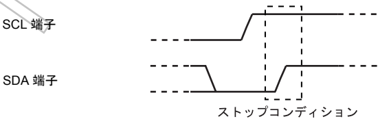
図 16-6 ストップコンディションの発生
