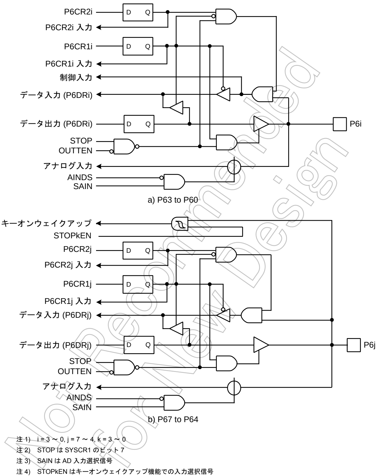
図 5-8 P6 ポート
