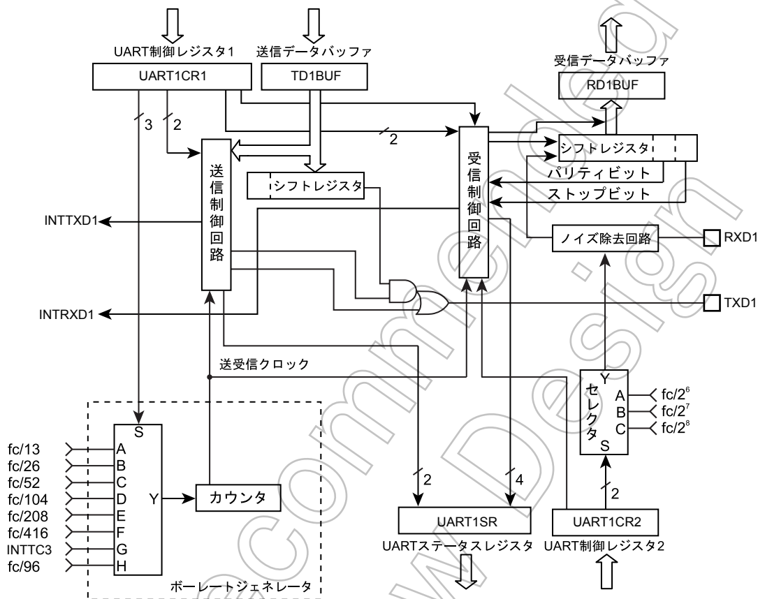
図 12-1 UART1 ( 非同期型シリアルインタフェース )
