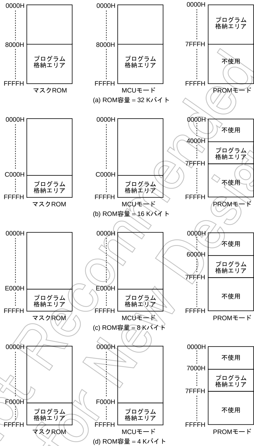
図 19-1 プログラム格納エリア
