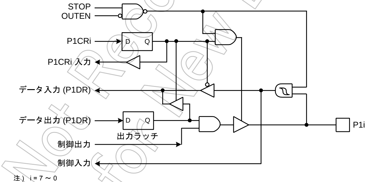
図 5-3 P1 ポート
