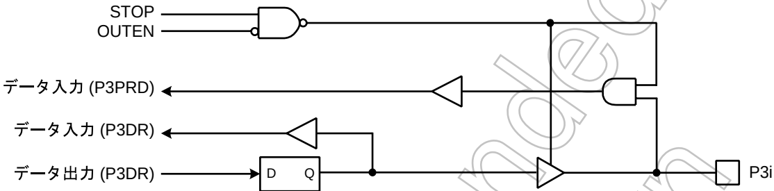
図 5-5 P3 ポート
