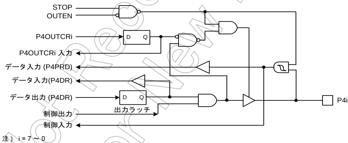
図 5-6 P4 ポート
