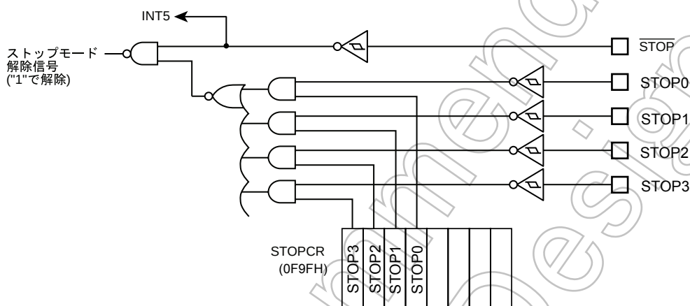
図 18-1 キーオンウェイクアップ回路
