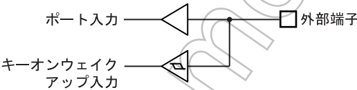
図 18-2 キーオンウェイクアップ入力とポート入力
