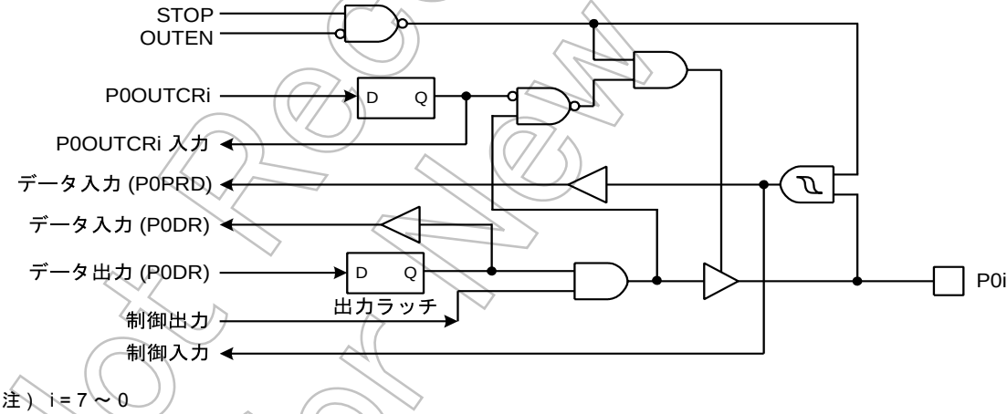
図 5-2 P0 ポート
