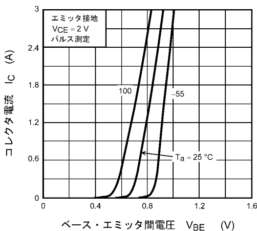
図 7.5 I_C - V_{BE}
