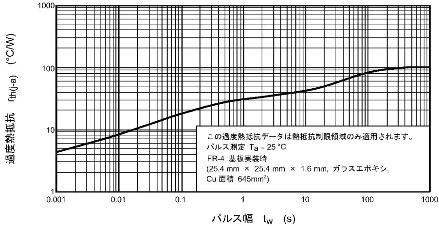
図 7.6 r_{th(j-a)} - t_w (最大値 (保証値))
