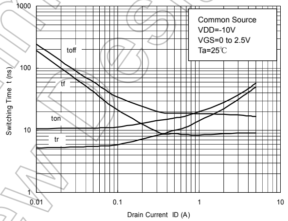
t - ID
