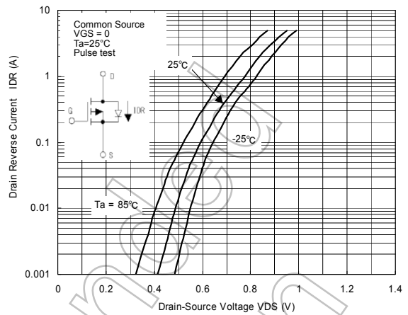
IDR - VDS
