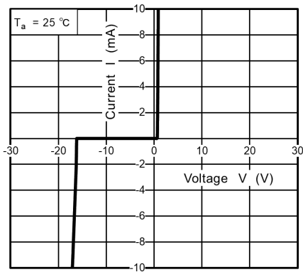
Fig. 7.1 I - V
