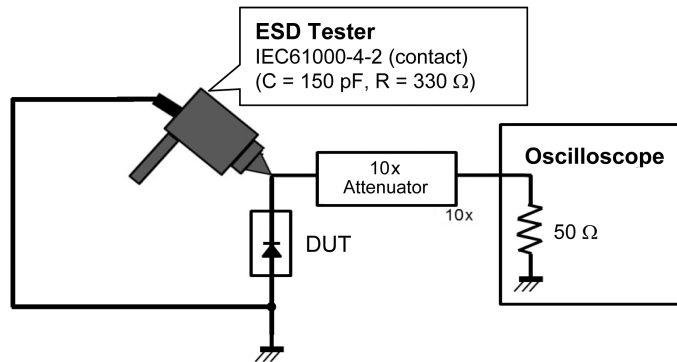
Fig. 9.3 IEC61000-4-2 (Contact)
