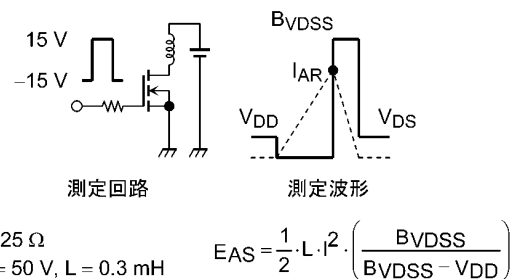
図 8.16 測定回路/測定波形
