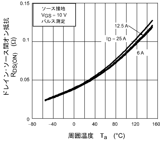
図 8.7 R_{DS(ON)} - T_a
