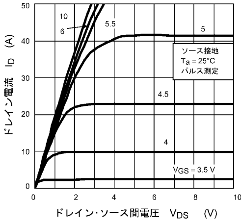
図 8.1 I_D - V_{DS}
