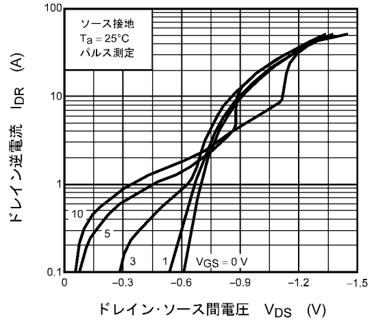
図 8.8 I_{DR} - V_{DS}
