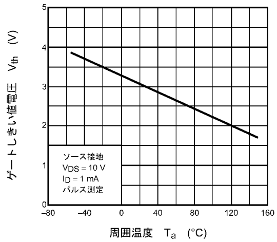
図 8.10 V_{th} - T_a
