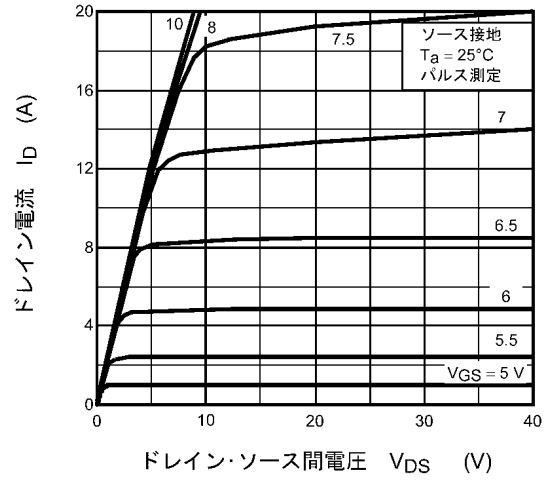
図 8.2 I_D - V_{DS}
