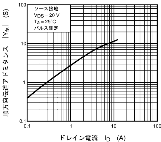
図 8.5 |Y_{fs}| - I_D
