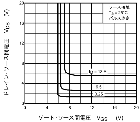
図 8.4 V_{DS} - V_{GS}
