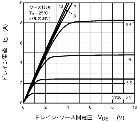
図 8.1 I_D - V_{DS}
