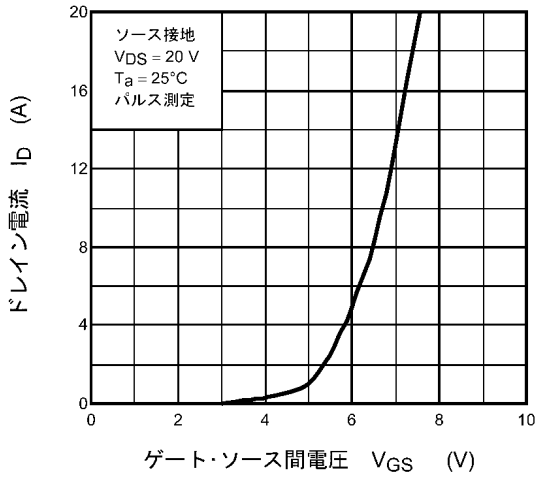
図 8.3 I_D - V_{GS}
