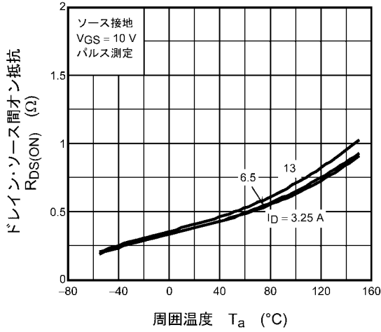
図 8.7 R_{DS(ON)} - T_a
