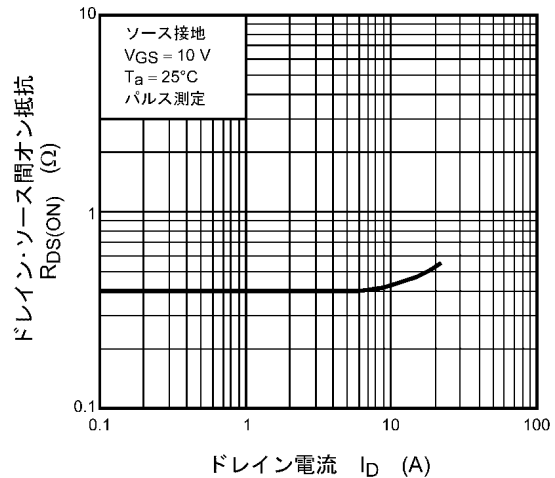
図 8.6 R_{DS(ON)} - I_D
