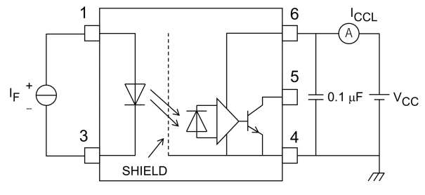
図 12.1.4 ICCL測定回路
