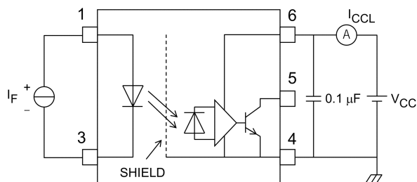
図 12.1.4 I CCL 測定回路
