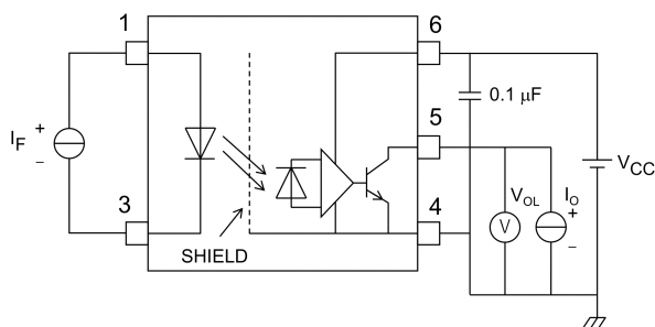
図 12.1.2 V OL 測定回路
