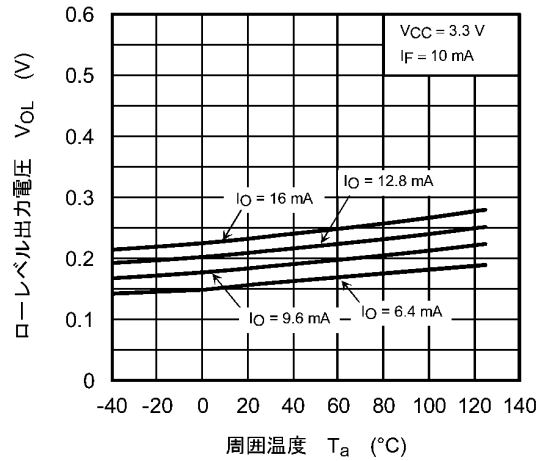
図 12.2.4 V_{OL} - T_a
