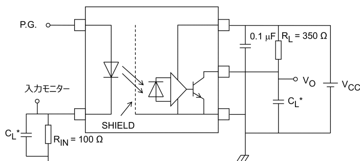
図 12.1.5 伝搬遅延時間測定回路, 波形
