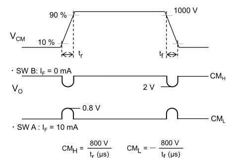
図 12.1.6 コモンモード過渡耐性測定回路, 波形
