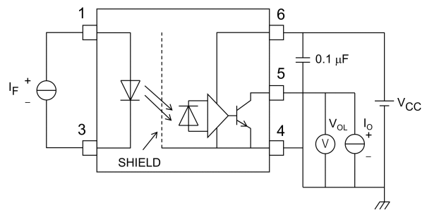
図 12.1.2 VOL測定回路
