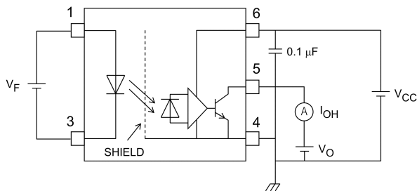
図 12.1.1 IOH測定回路
