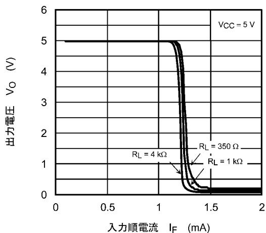
図 12.2.5 V_O - I_F
