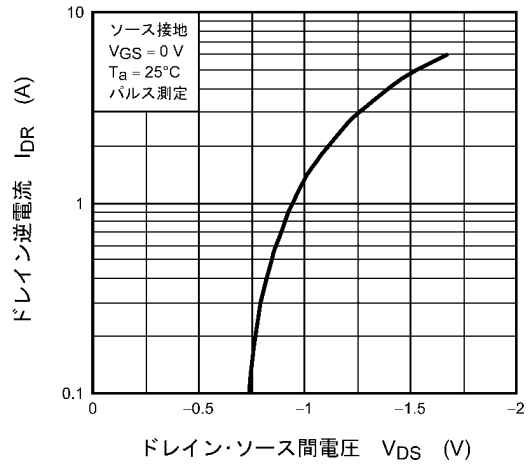
図 8.8 I_{DR} - V_{DS}
