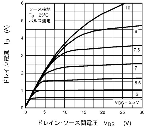
図 8.2 I_D - V_{DS}
