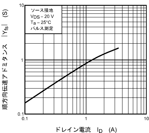
図 8.5 |Y_{fs}| - I_D
