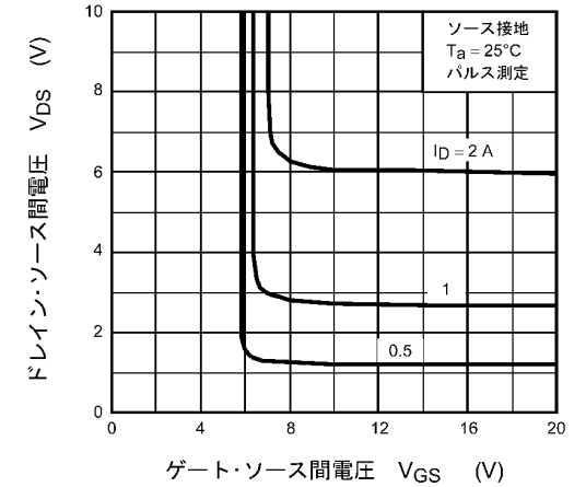
図 8.4 V_{DS} - V_{GS}
