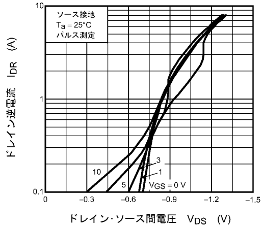
図 8.8 I_{DR} - V_{DS}
