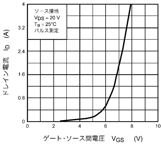
図 8.3 I_D - V_{GS}
