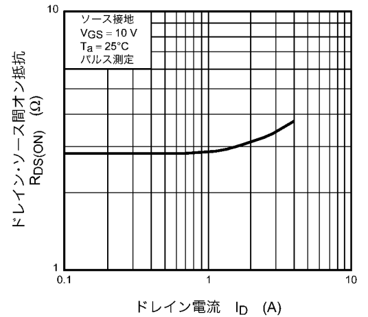
図 8.6 R_{DS(ON)} - I_D
