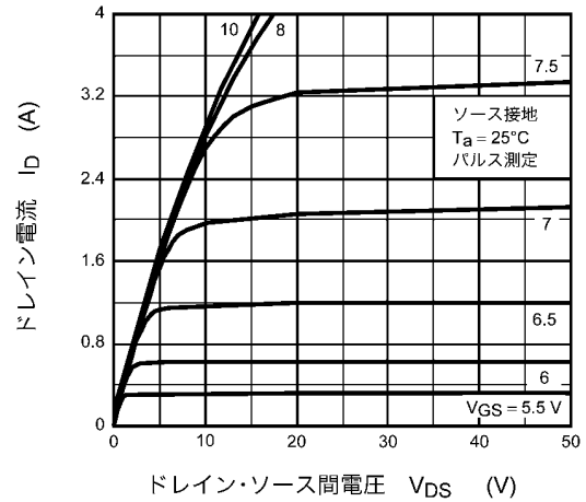
図 8.2 I_D - V_{DS}
