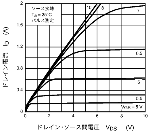
図 8.1 I_D - V_{DS}
