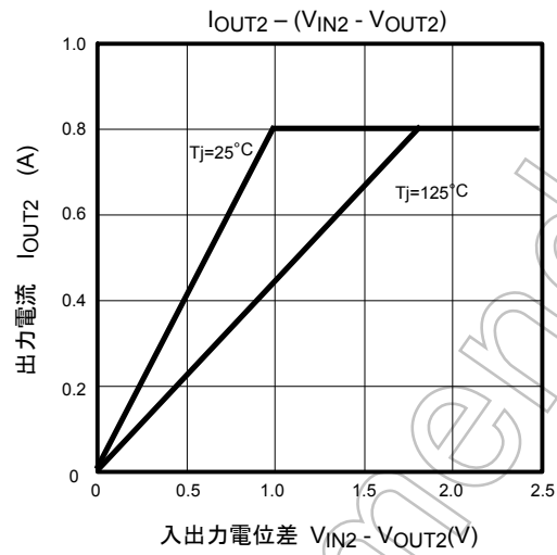
図6 最小入出力電位差
