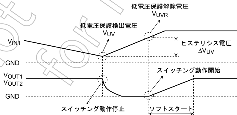
図 8 低電圧保護動作
