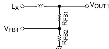
図3 出力電圧設定抵抗
