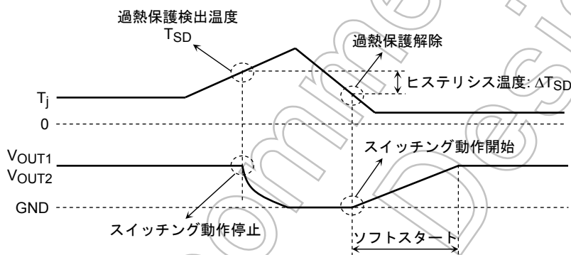
図 7 過熱保護動作
