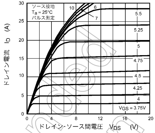
図 8.2 I_D - V_{DS}
