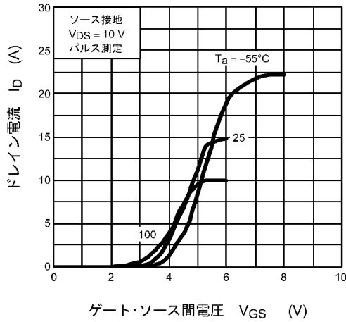
図 8.3 I_D - V_{GS}
