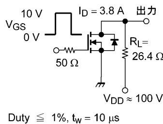
図 6.2.1 スwitching時間の測定回路例
