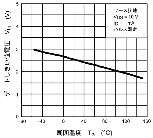
図 8.10 V_{th} - T_a
