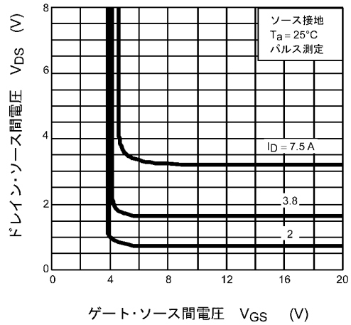
図 8.4 V_{DS} - V_{GS}
