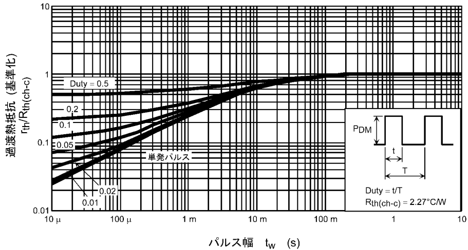
パルス幅 t_w (s) 図 8.13 r_{th}/R_{th(ch-c)} - t_w (最大値 (保証値))
