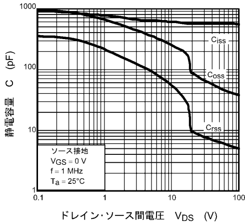
図 8.9 C - V_{DS}
