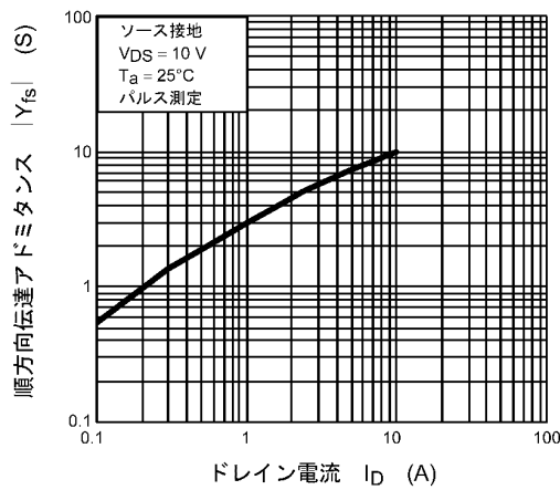
図 8.5 |Y_{fs}| - I_D
