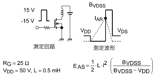
図 8.16 測定回路/測定波形
