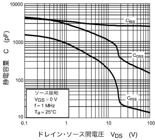
図 8.9 C - V_{DS}
