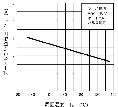
図 8.10 V_{th} - T_a
