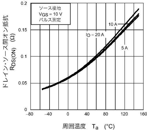
図 8.7 R_{DS(ON)} - T_a
