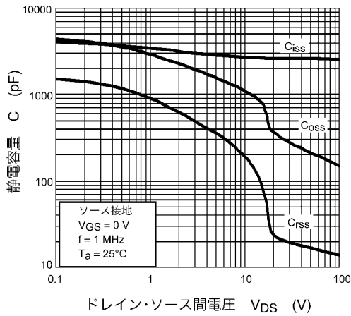
図 8.9 C - V_{DS}
