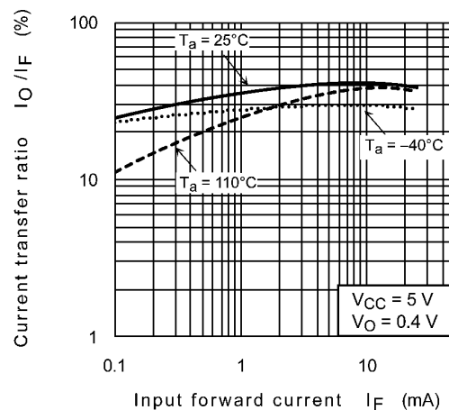
Fig. 12.2.4 I_O/I_F - I_F
