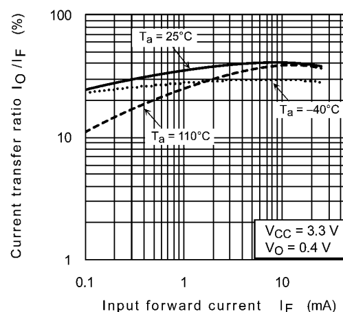
Fig. 12.2.6 I_O/I_F - I_F
