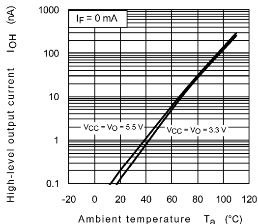
Fig. 12.2.2 I_{OH} - T_a
