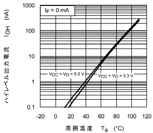
図 12.2.2 I_{OH} - T_a
