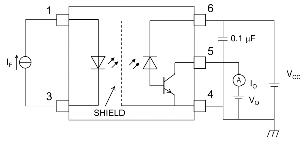
図 12.1.4 I O 測定回路
