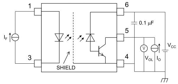
図 12.1.2 V OL 測定回路
