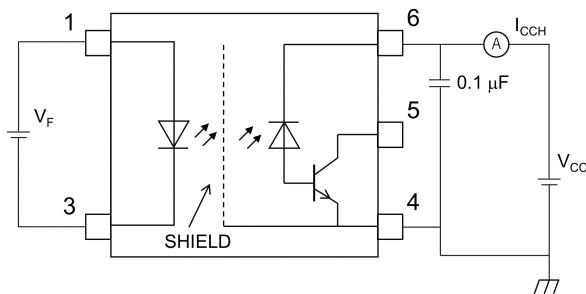
図 12.1.3 I CCH 測定回路
