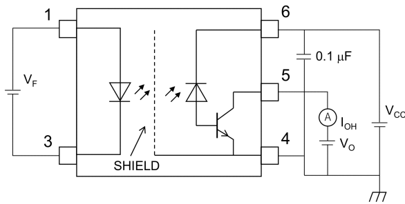
図 12.1.1 I OH 測定回路
