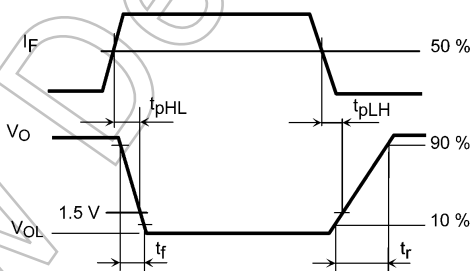
図 12.1.5 伝搬遅延時間測定回路, 波形
