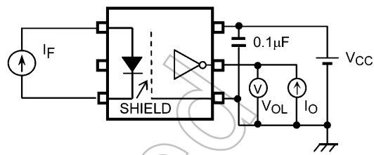
図 12.1.2 VOL測定回路
