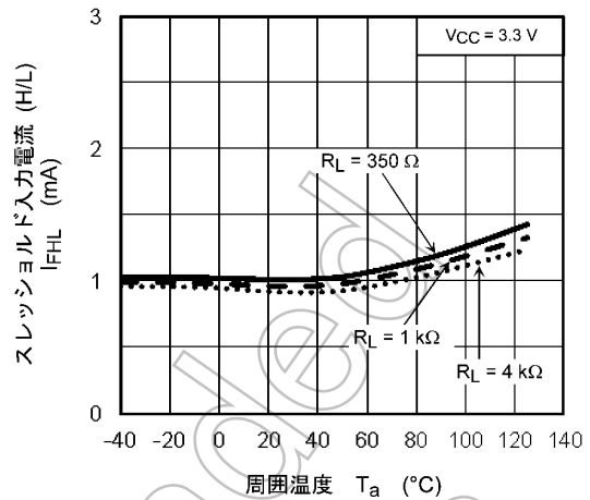
図 12.2.8 I_{FHL} - T_a
