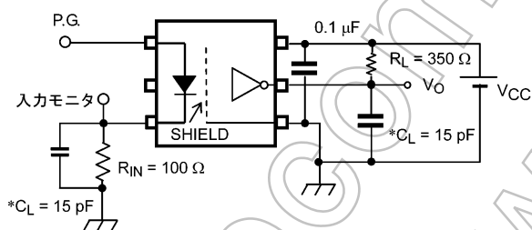
図 12.1.5 伝搬遅延時間測定回路, 波形
