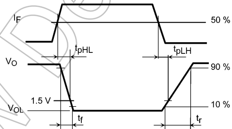
図 12.1.5 伝搬遅延時間測定回路, 波形
