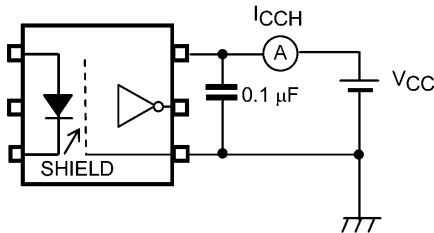
図 12.1.3 I CCH 測定回路
