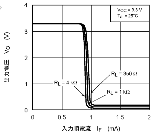
図 12.2.6 V_O - I_F
