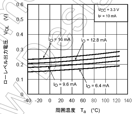
図 12.2.4 V_{OL} - T_a
