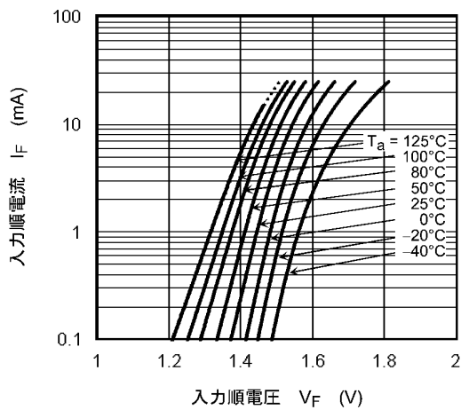
図 12.2.1 I_F - V_F
