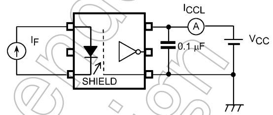
図 12.1.4 I CCL 測定回路
