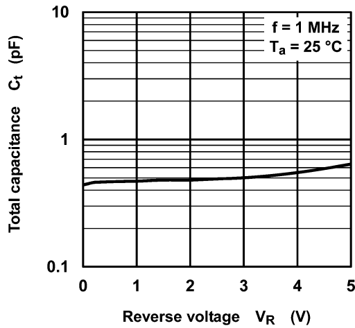
Fig. 7.3 C t - V R
