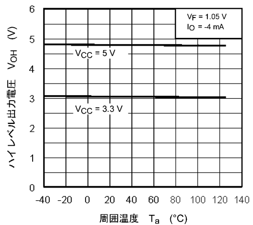
図 12.2.4 V_{OH} - T_a
