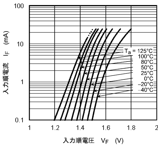
図 12.2.1 I_F - V_F
