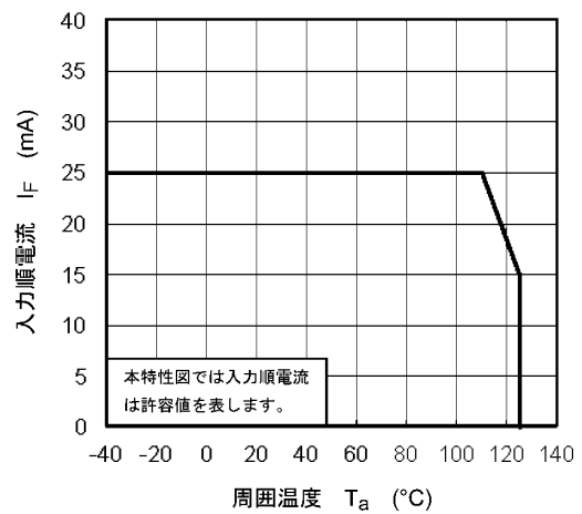
図 12.2.2 I_F - T_a
