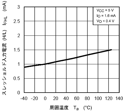
図 12.2.7 I_{FHL} - T_a
