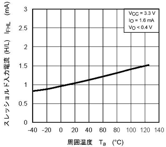
図 12.2.8 I_{FHL} - T_a
